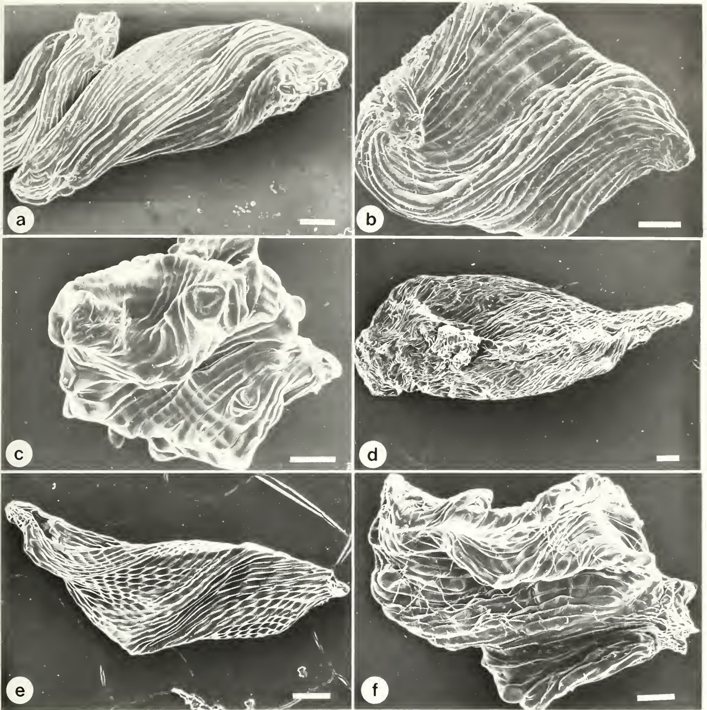
FIGURE 5.—Seeds of Kohleria (scale length = 50 \mu m): a, K. neglecta ; b, K. amabilis var. bogotensis ; c, K. diastemoides ; d, K. grandiflora ; e, K. hirsuta var. hirsuta ; f, K. inaequalis var. inaequalis . Micrograph a of García-Barriga 10737 (US); b of Purdie s.n. (K); c of Lehmann 8892 (NY); d of Cuatrecasas 11683 (US); e of Barkley 35221 (NY); f of Lehmann 1236 (NY).
