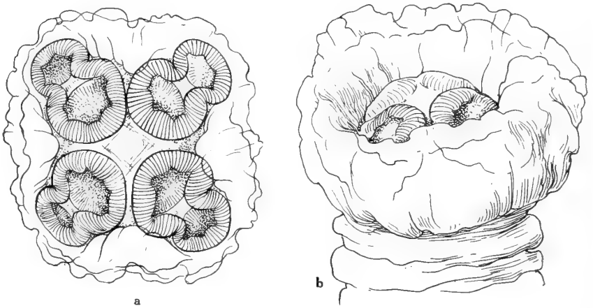
FIG. 3. Scolex vom Amphoteromorphus peniculus Diesing. a, Scolex von vorn gesehen; b, von der Seite.
