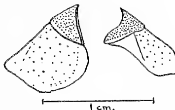
Fig. 12.— M. adelicana . Mandibles.
