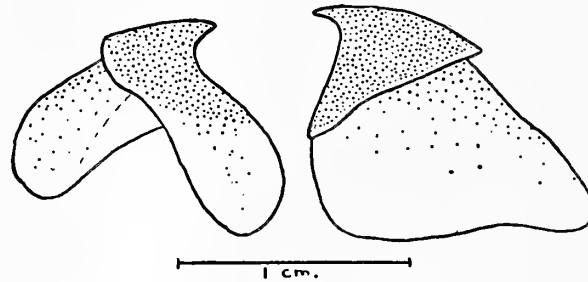
Fig. 8.— M. albida . Mandibles.
