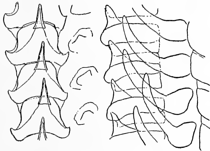
Fig. 20.— M. aurora . Radula.
