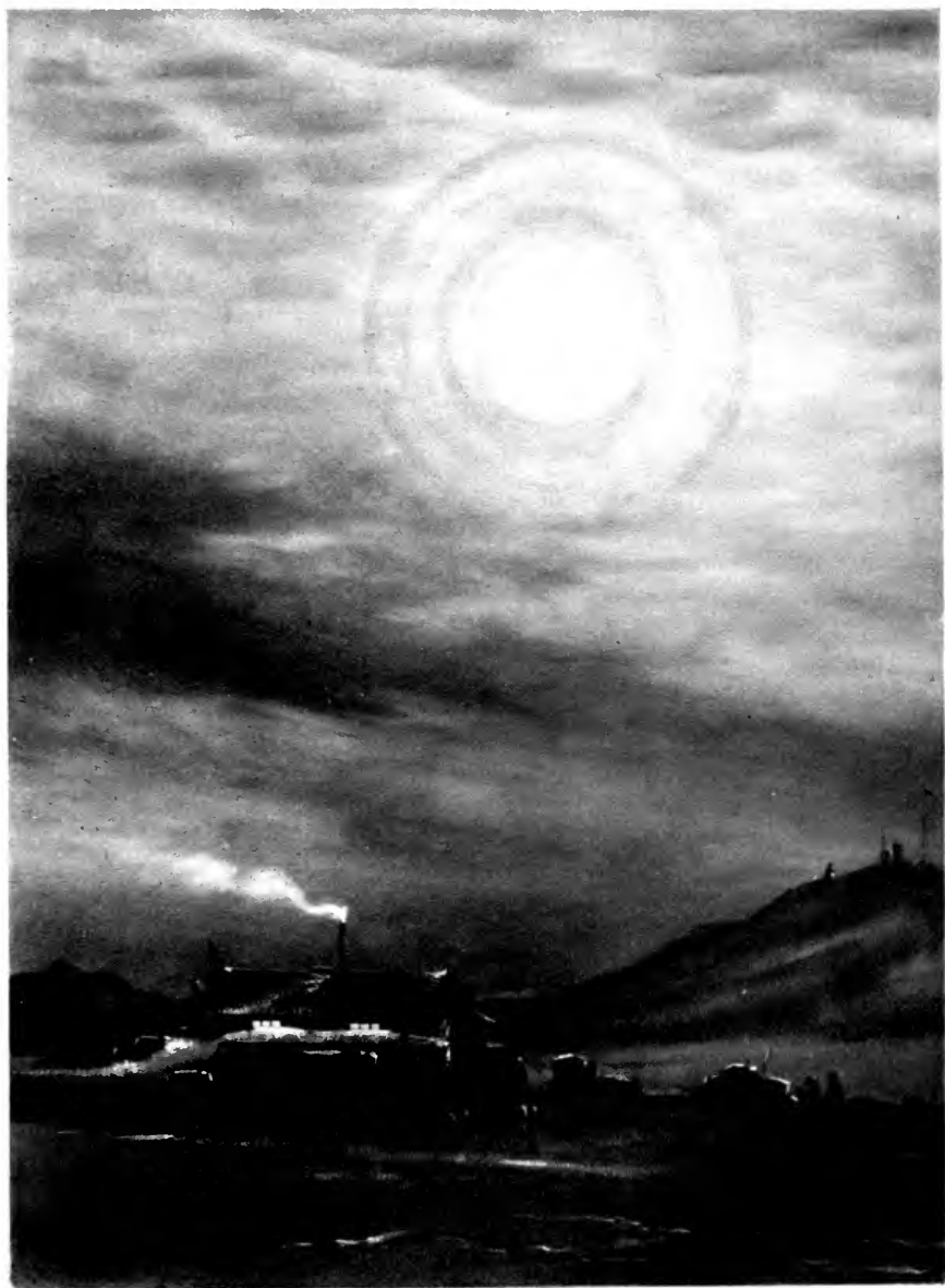
LUNAR CORONA.
