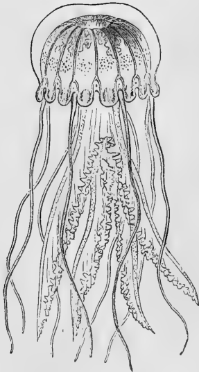
FIG. 20.—JELLY-FISH ( Pelagia cyanella , Agassiz).
