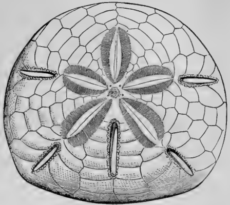
FIG. 29.—KEY-HOLE-URCHIN ( Mellita quinquefora , Agassiz).
