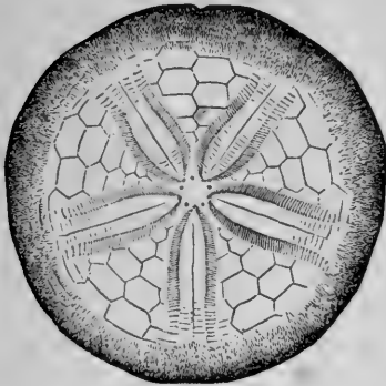
FIG. 28.—CAKE-URCHIN ( Echinarachnius parma , Gray).
