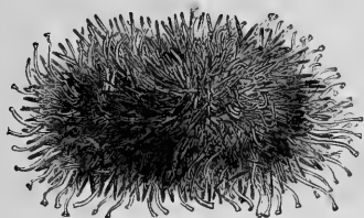
FIG. 26.—SEA-URCHIN ( Toxoneustes dробachien-sis , Agassiz).
