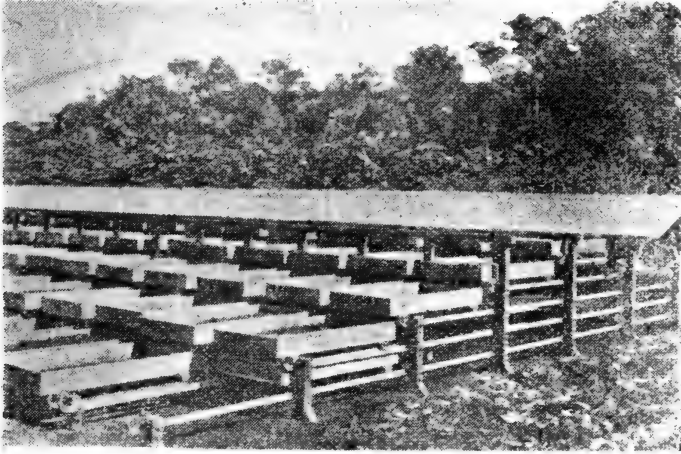
圖 207 特殊的日曬乾燥設備
