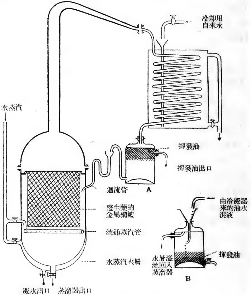
圖 190 揮發油蒸溜裝置
