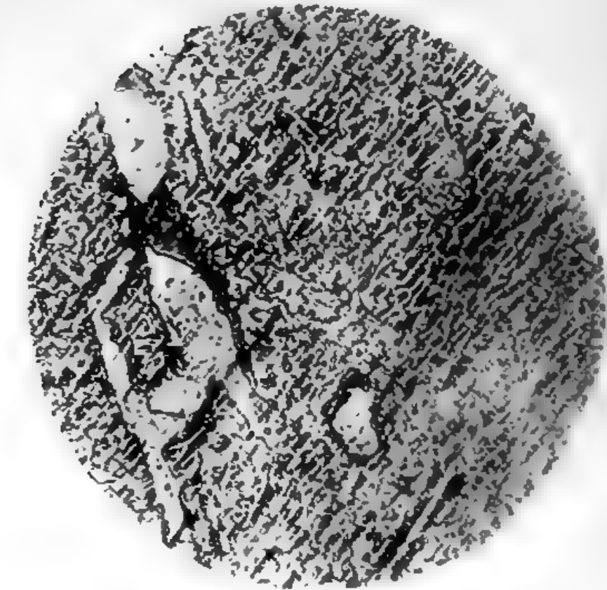
7. Morradal Ni. - 18.77% Vergr. 420
