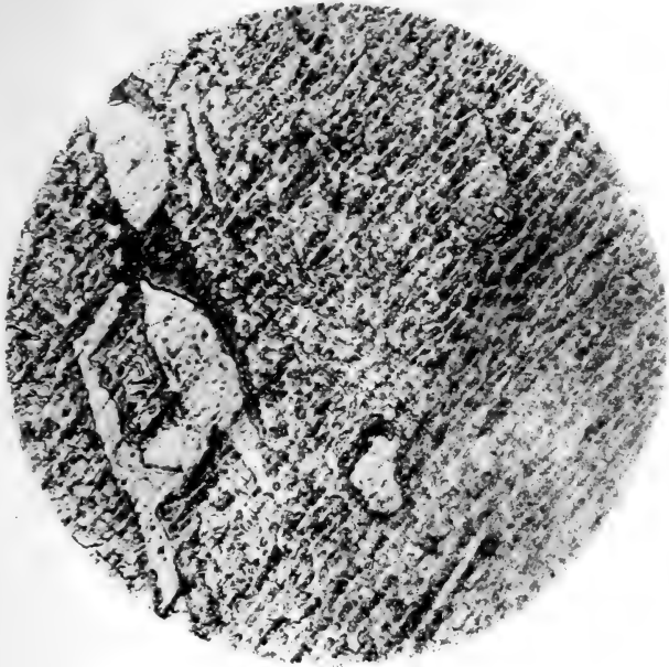
7. Morradal Ni - 18.77% Vergr. 420
