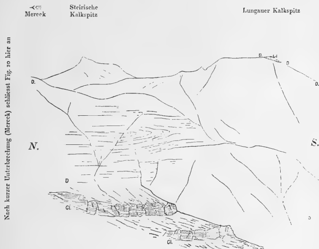
Fig. 11. Eingefalteter, scheinbar flach lagernder Diploporendolomit ( D ) zwischen der Masse des Glimmerschiefers ( Gl ) am Fusse der Berge und dem Denudationsrest desselben Gesteins auf dem Gipfel der Lungauer Kalkspitz.
