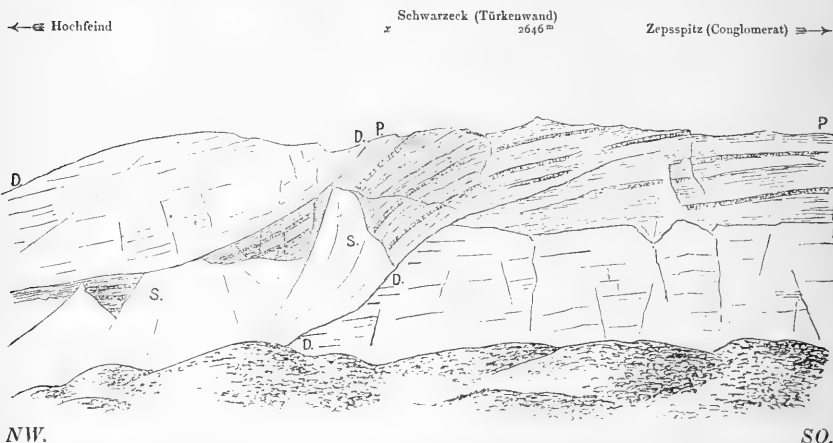
Fig. 7. Der Pyritschiefer (P.) bildet am Schwarzeck eine steil gestellte, unregelmässige Syncline zwischen zwei aus Dolomit bestehenden Zügen und setzt den NW.—SO. streichenden Hauptkamm (Mitte und SO.-Hälfte des Bildes) zusammen. Der Dolomit (D.) bildet einen nach SW. abzweigenden Nebenkamm (← Hochfeind), unter den in Folge unregelmässiger Verquetschung der Pyritschiefer (bei x) einschiesst. In Vordergrund Moränenhügel. Links Schutt (S.). Während des Aufstiegs zum Gipfel gezeichnet.
