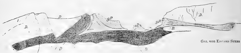
Fig. 3. Eingefaltete Pyritschiefer (P. schwarzer Pyritschiefer, gP. gelber Pyritschiefer mit Glimmerblättchen) im Dolomit (D). »Am Thor« vom Zehnerkar.
