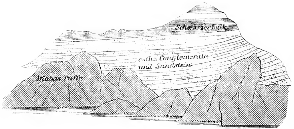
Am Isker bei Obletnja.
