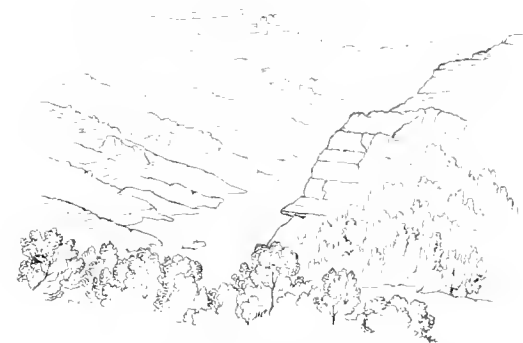
Isker in Gebiete der rothen Conglomerats oberhalb Čerepić . • Schieferige Quarzite . → Kalkberge des Vraca Balkan .
