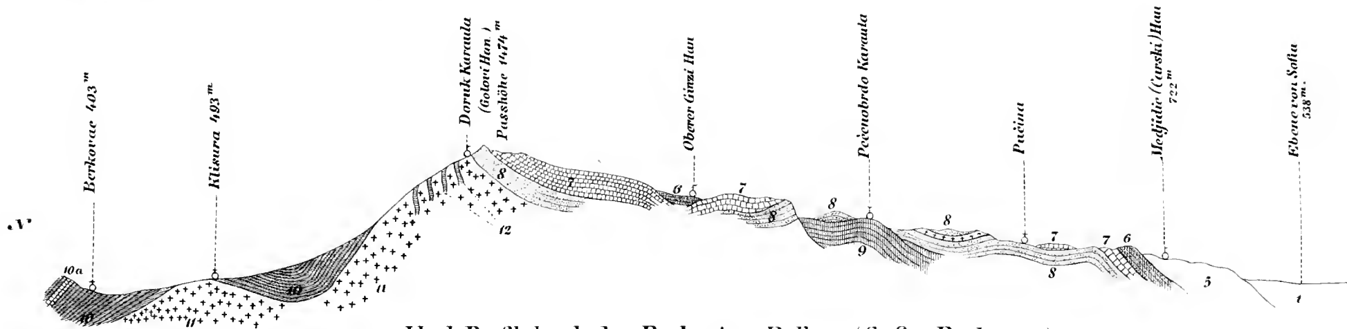
Ideal Profil durch den Berkovica Balkan (Sofia-Berkovae).
