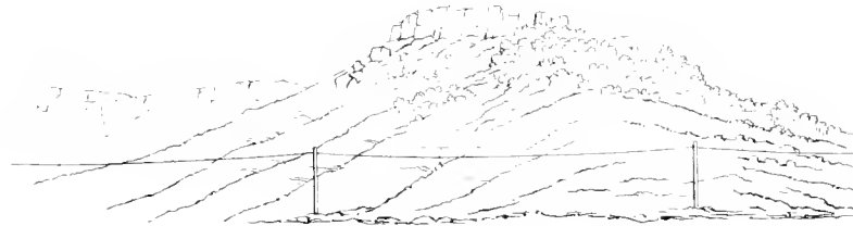
Stuhlberge beim Günei Han .
