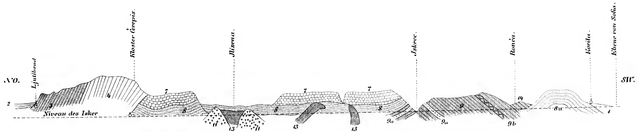
Ideal Profil von Sofia nach Ljutibrod am Isker.
