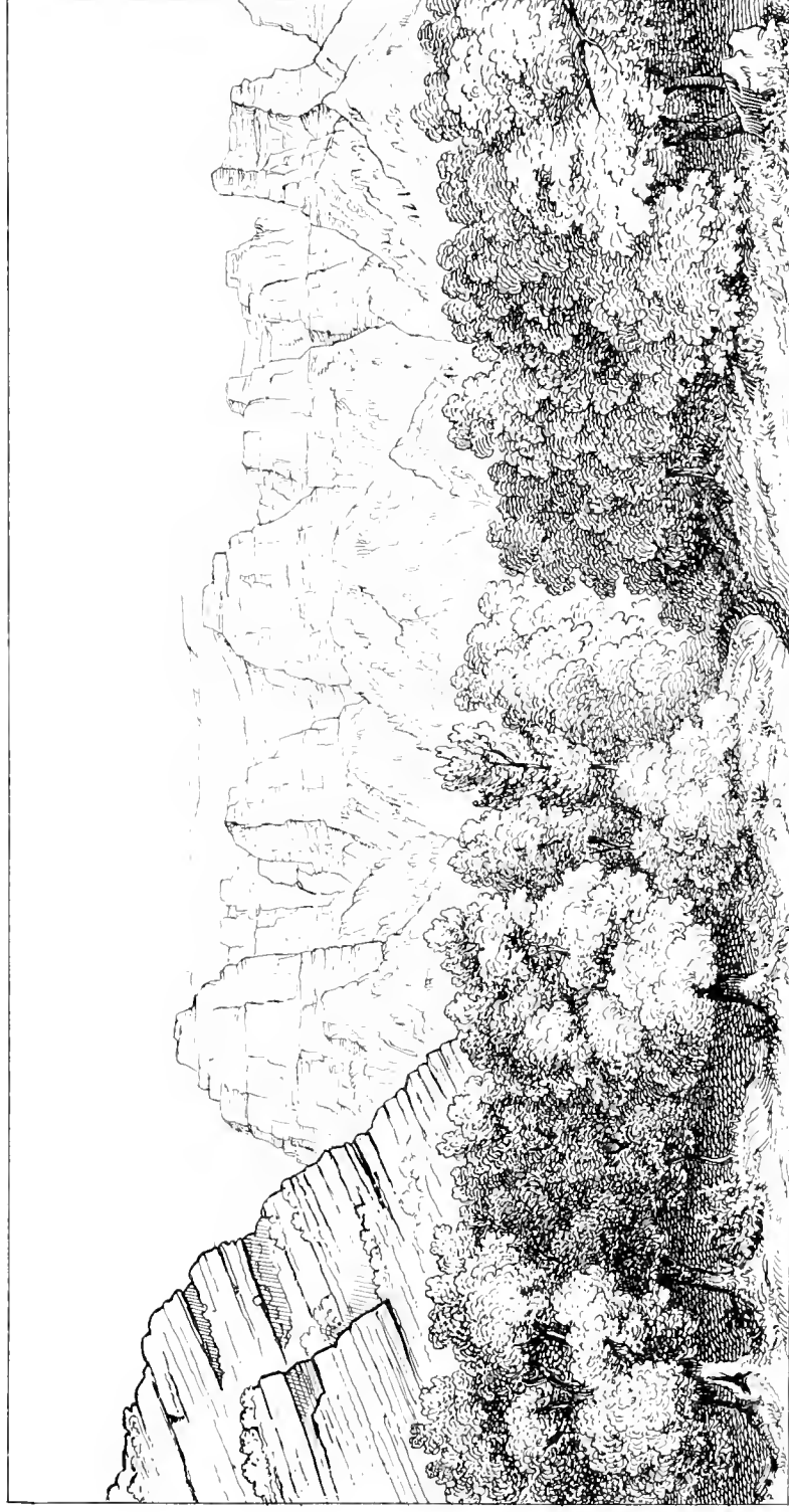
Hintergrund der Schlucht von Obletnja ( Südfall des Traca Balkan. )
