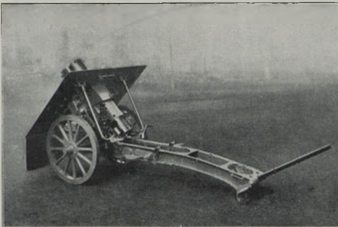
10 cm horská houfnice vzor 16 (Škoda).
