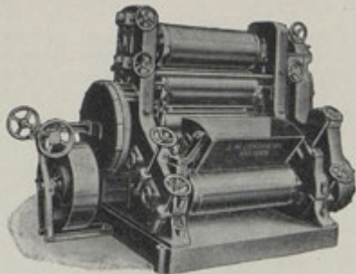
Podélný třecí stroj.
