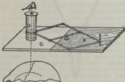
Dioptrograf k obkreslení lebky: G diopter, G skle- něná plocha, B prkno, S pisadlo.
