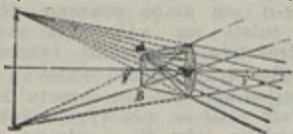
Obr. 1. Virtuální obraz u spojky.
