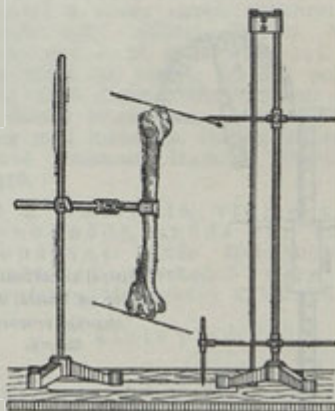
Parallelograf, sloužící k zjištění torse nadlokti.
