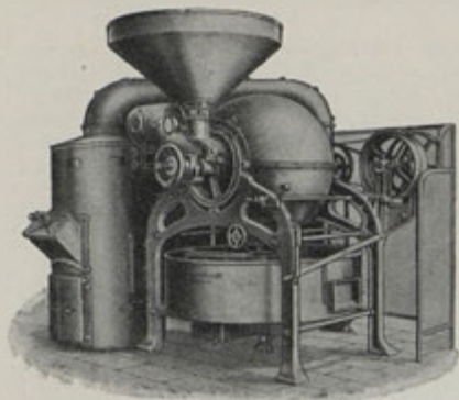
Pražič horkým vzduchem.
