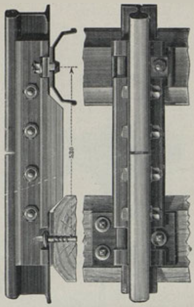
Spojení kolejnic.
