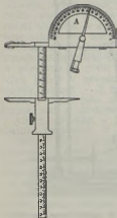
Přístroj ku měření proporcí na kostře. A zachycuje proporce úhlové.
