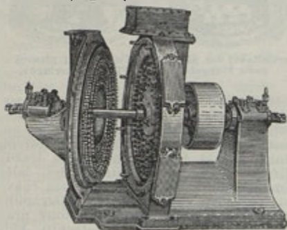
Desintegrátor Kruppův.
