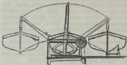
Davit kvadrantový.
