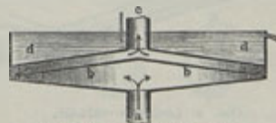
Obr. 7. Pistoriova pánev.
