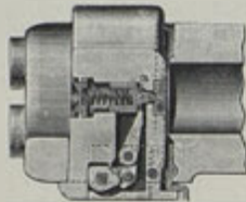
Vodorovný řez středem závěru; a) úterník.
