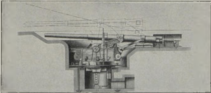
Pobřežní dělo se sklápěcí lafetou (Krupp).
