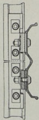
Kolejnice na železném pražci.
