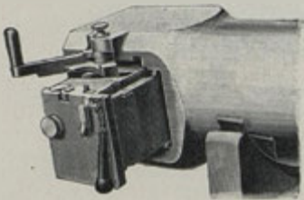
Pohled z prava, závěr otevřen.
