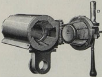
Pohled ze zadu, závěr otevřen.
