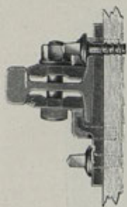
Průřez kolejnice s rámovými pražci.
