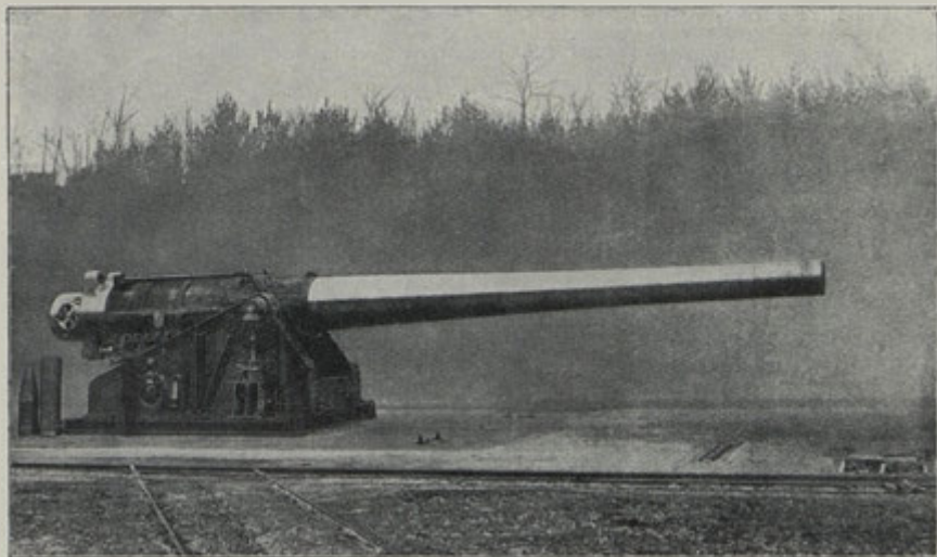
Dalekonosné dělo, 85 cm L/45 (Škoda).
