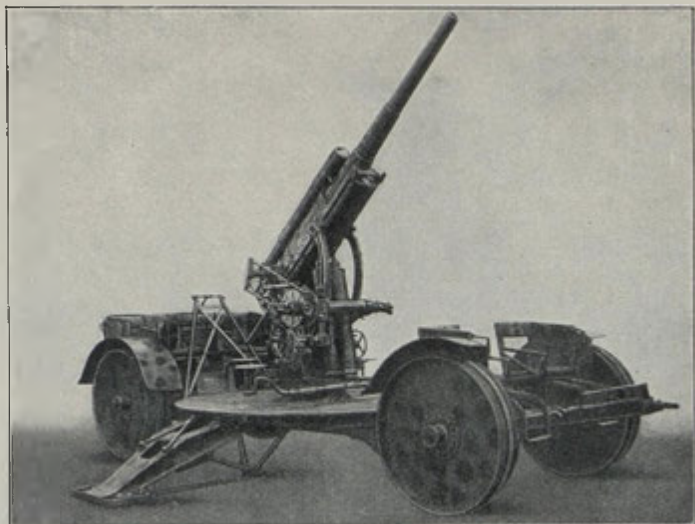
8.8 cm mot. dělo protiletadlové s otáčecí lafetou.
