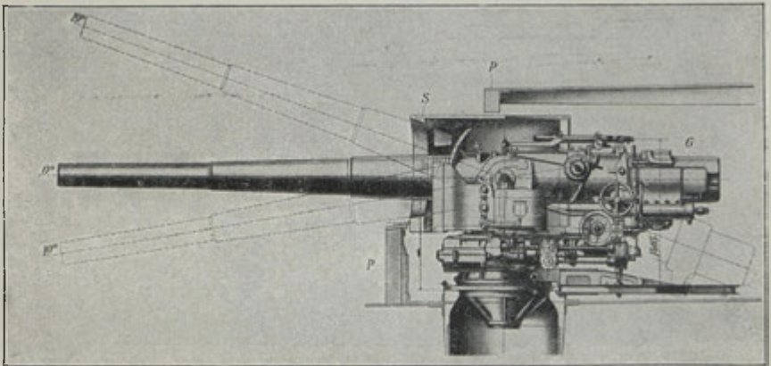
15 em pevnostní dělo (Krupp). P = pancéř kaseňat, G = dělo, S = kul. štít.
