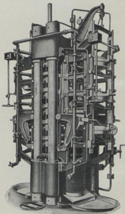
Hydraulický lis.
