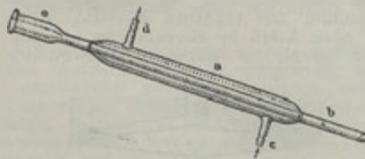
Obr. 4. Liebigův chladič.
