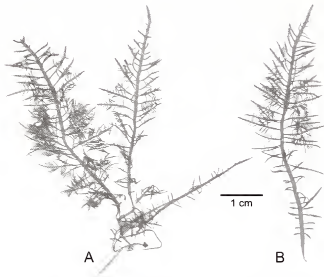
FIGURE 157. Pterocliadiella capillacea : A, B. Habits (JN-4611b, US Alg. Coll.-159295).
