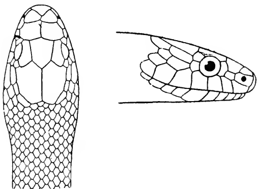
FIG. 27 (after Sordelli)
