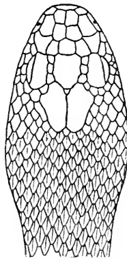
FIG. 35 (after Sordelli)
