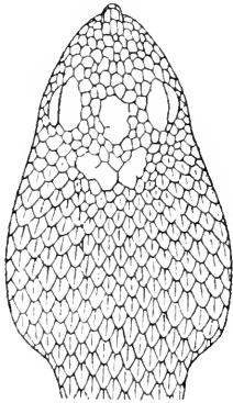
FIG. 38 (after Sordelli)
