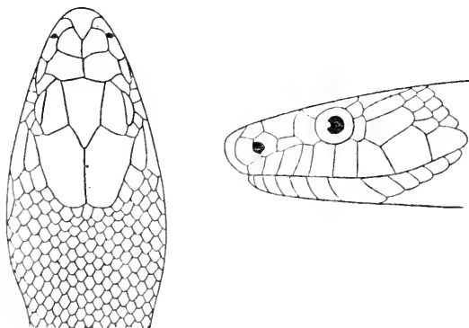
FIG. 26 (after Sordelli)
