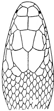
FIG. 22 (after Sordelli)
