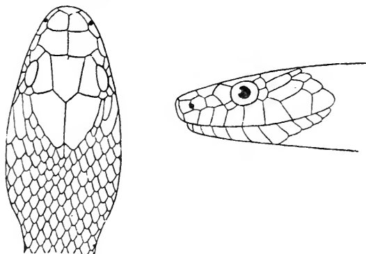
FIG. 23 (after Sordelli)
