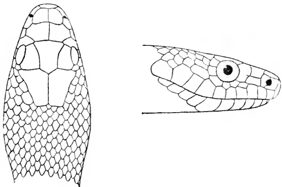
FIG. 21 (after Sordelli)
