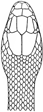
FIG. 29 (after Sordelli)
