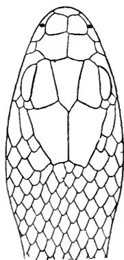
FIG. 19 (after Sordelli)
