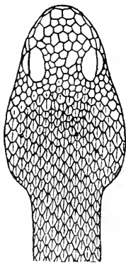
FIG. 36 (after Sordelli)
