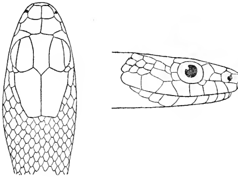
FIG. 20 (after Sordelli)
