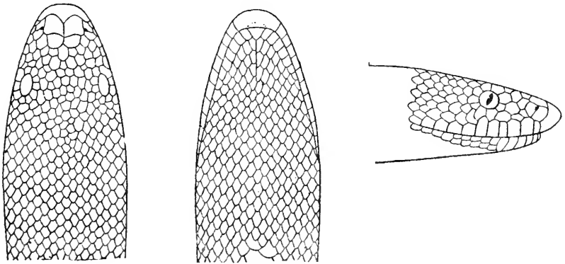
FIG. 15 (after Sordelli)
