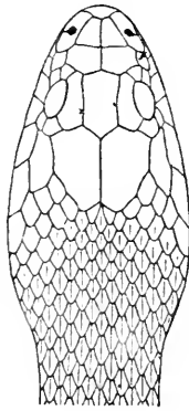
FIG. 18 (after Sordelli)
