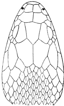
FIG. 16 (after Sordelli)
