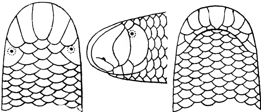
FIG. 14 (after Sordelli)
