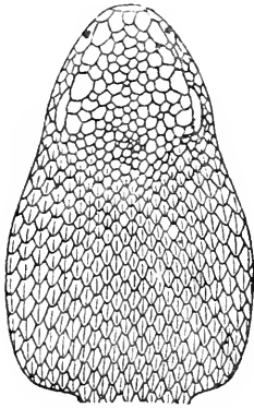
FIG. 41 (after Sordelli)
