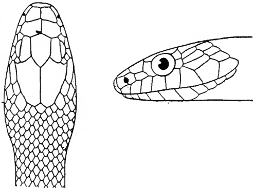
FIG. 28 (after Sordelli)
