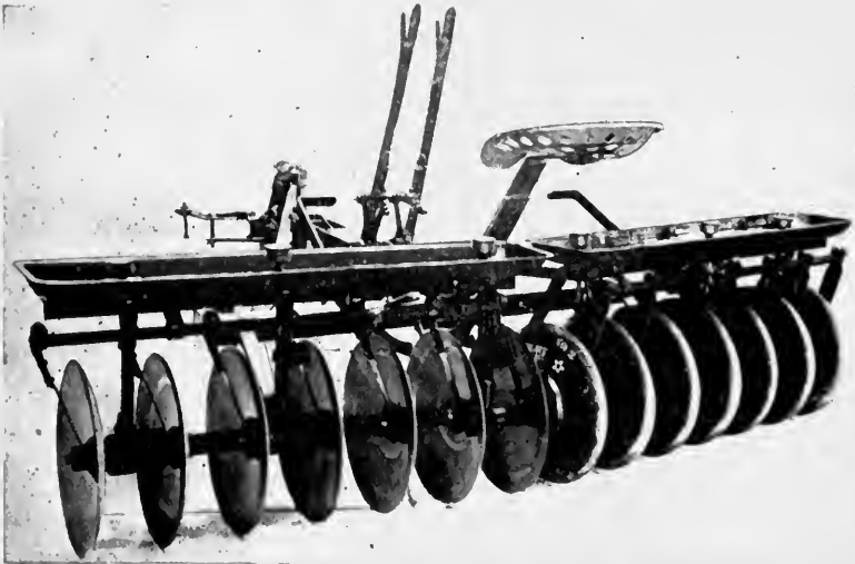
FIG. 148.—The solid disk.
