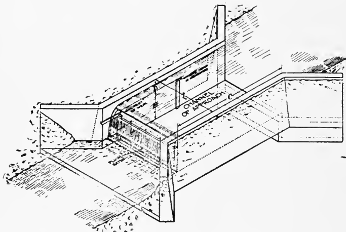
FIG. 120.—Rectangular weir.
