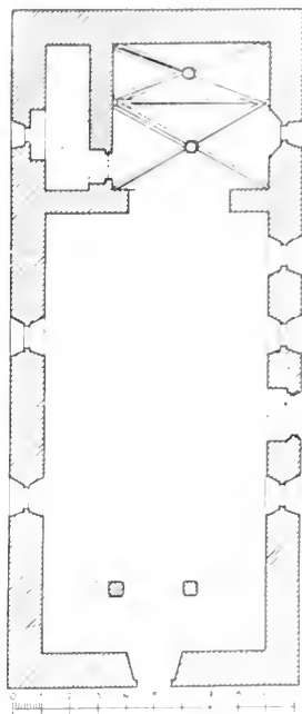
Obr. 191. Sulislav. Kostel sv. Vavřince. Půdorys.
