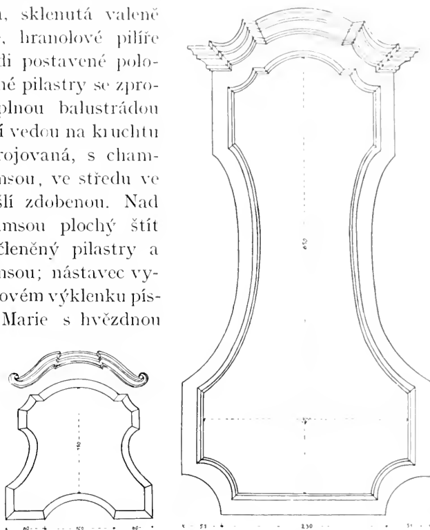
Obr. 140 Stříbro. Kostel Věch Svátých. Schema oken v boční a hlavní lodi.
