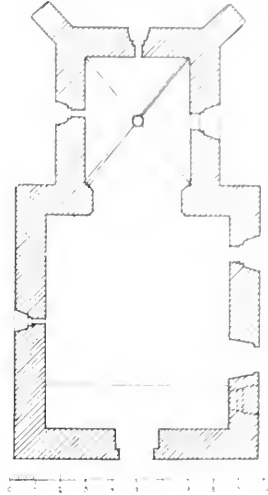
Obr. 184. Stříbro, Kostel sv. Petra. Půdorys.
