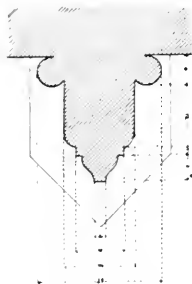
Obr. 73. Kladruby. Kláštr chrám. Profil triumf. oblouku v hrobce.
