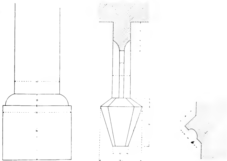
Obr. 137.—138. Stříbro. Kostel Všeoh Svatý h. Operák kněžiště. Profil zebra s konsolou v přízemi a profil římsy v 1. patře věže.
