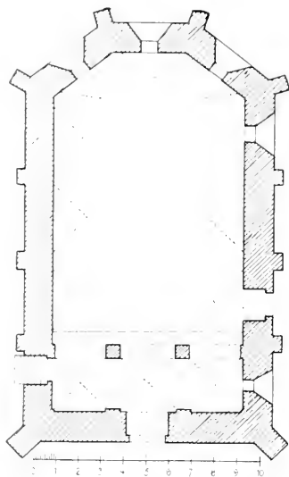
Obr. 156. Stříbro. Kostel P. Marie. Půdorys.
