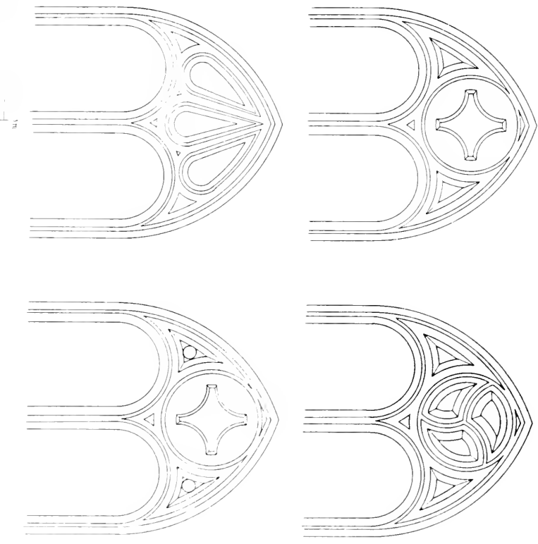
Obr. 30. Avenioy. Kostel sv. Barbary. Okenní kruzový v klenbě.
