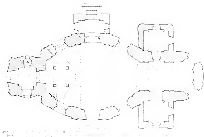
Obr. 93. Leštany. Kostel sv. Petra a Pavla. Půdorys.
