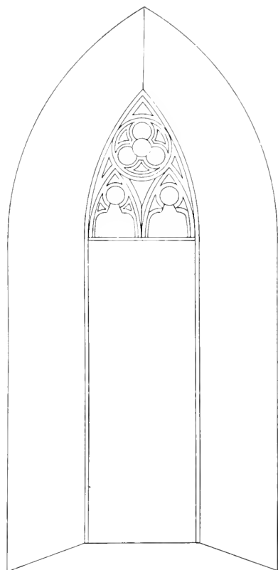
Obr. 188. Stříbro, Kostel sv. Petra. Okno v kněžišti.
