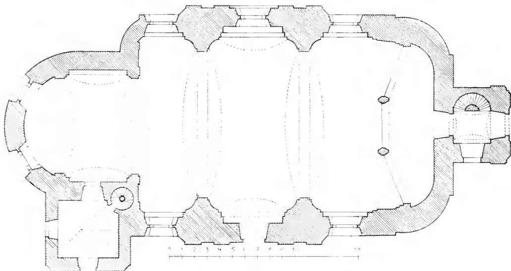
Obr. 207. Touškov n. Mží. Kostel sv. Jana Křt. Pudorys.
