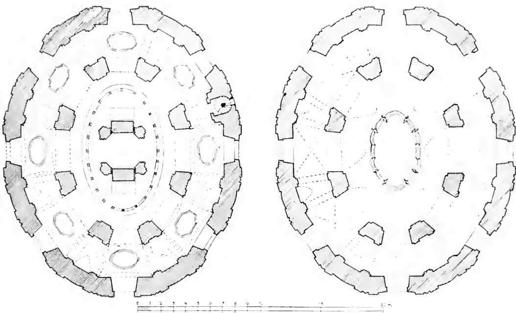
Obr. 10.—11. Dobruška. Kostel sv. Víta. Půdorys přízemí a ve výšší empor.
