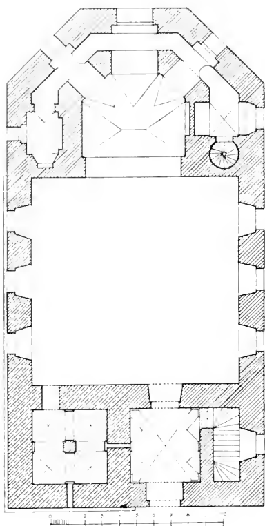
Obr. 197. Svojsín. Kostel sv. Petra a Pavla. Púdorys (bez hrobky).
