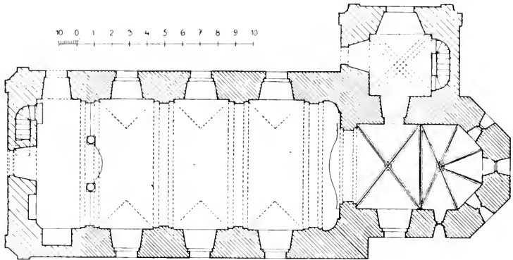
Obr. 105. Prostiboř. Kostel sv. Mikuláše. Púdorys.
