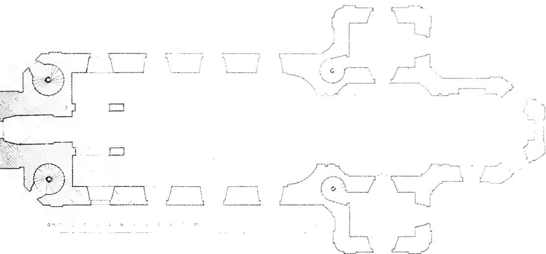
Obr. 38. Chotěšov. Kostel P. Marie. Půdorys.
