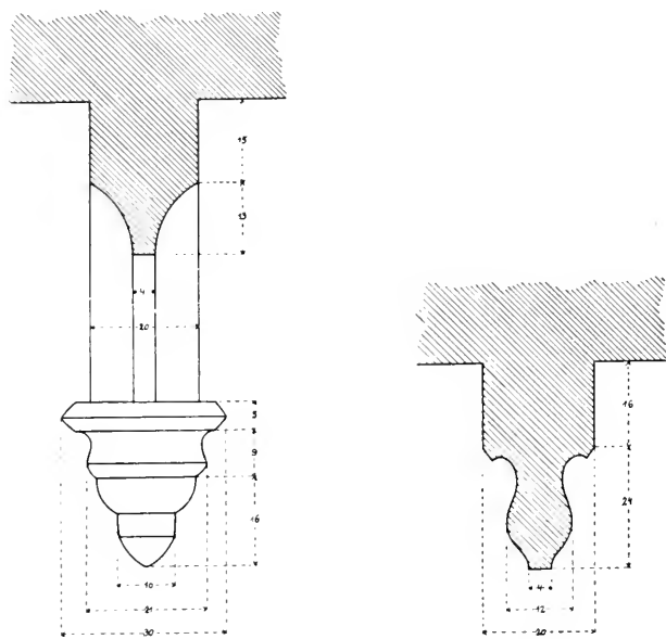
Obr. 89. Kostelec, Kostel sv. Jana Křtitele. Profil žebra a konsola v sakristii a profil žebra v kněžišti.
