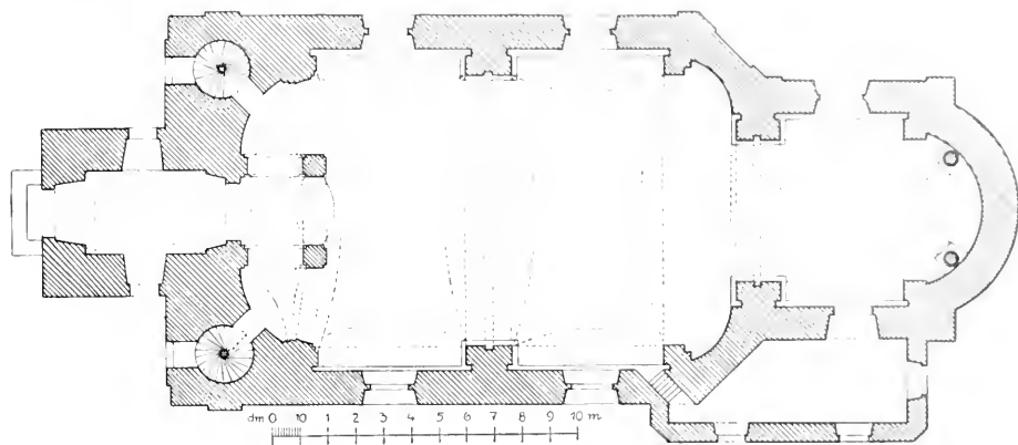
Obr. 112. Skapce, Kostel sv. Trojice, Pídrorys.
