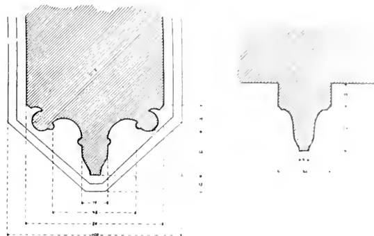
Obr. 231. Všeruby, Kostel sv. Ducha. Profil oblouku triumfálního a žebra v sakristii.
