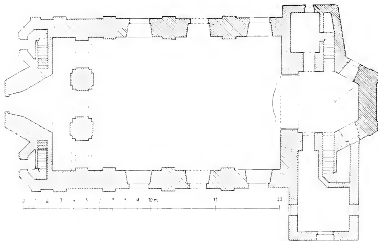
Obr. 235. Záchlumí, Kostel P. Marie, Pudorys.
