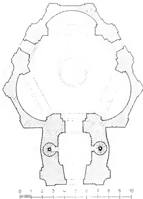
Obr. 101. Ostrov. Kostel sv. Václava. Půdorys.
