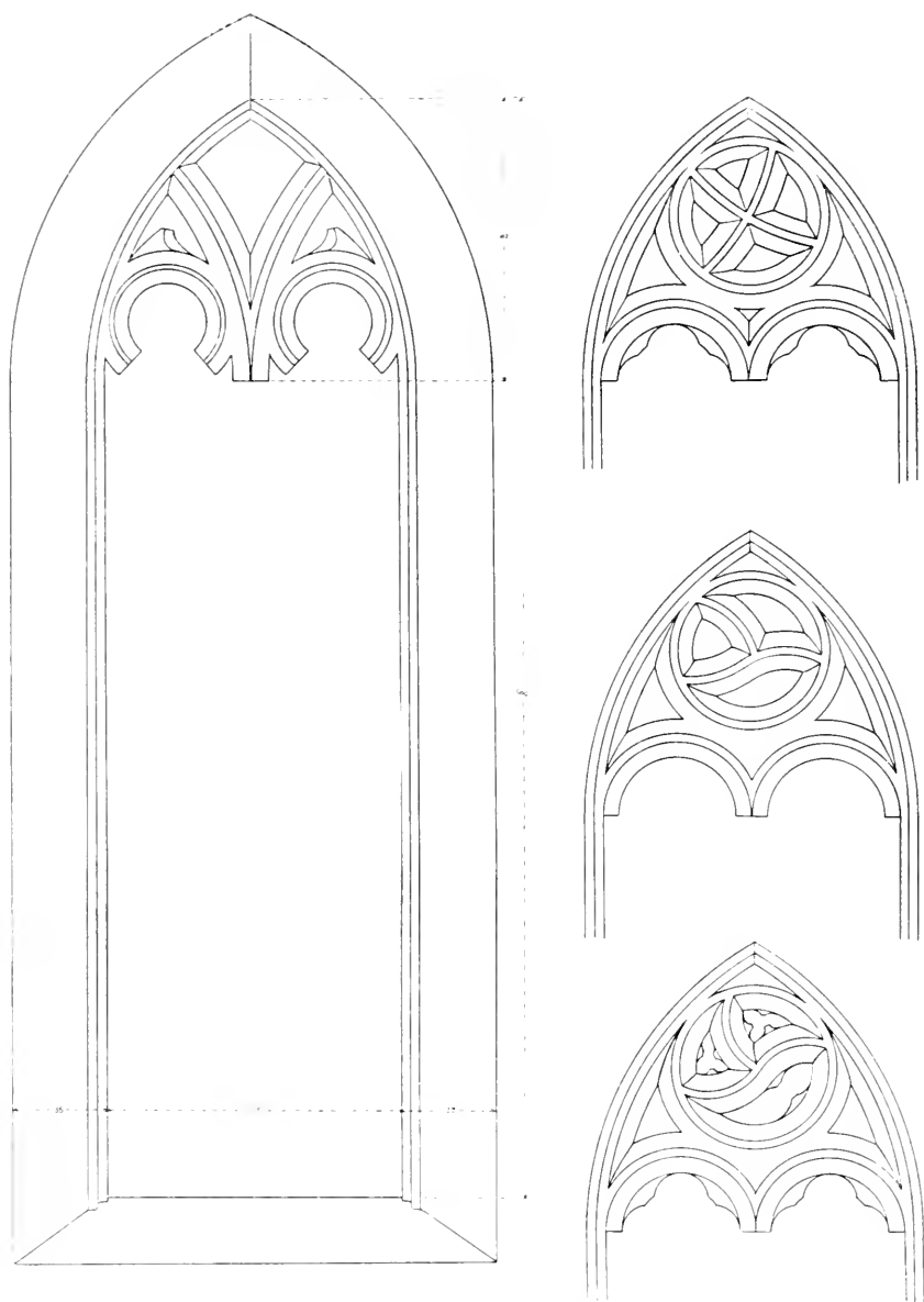
Obr. 139. Stříbro, Kostel Věch Svatých. Kruzby okenní ve věži.
