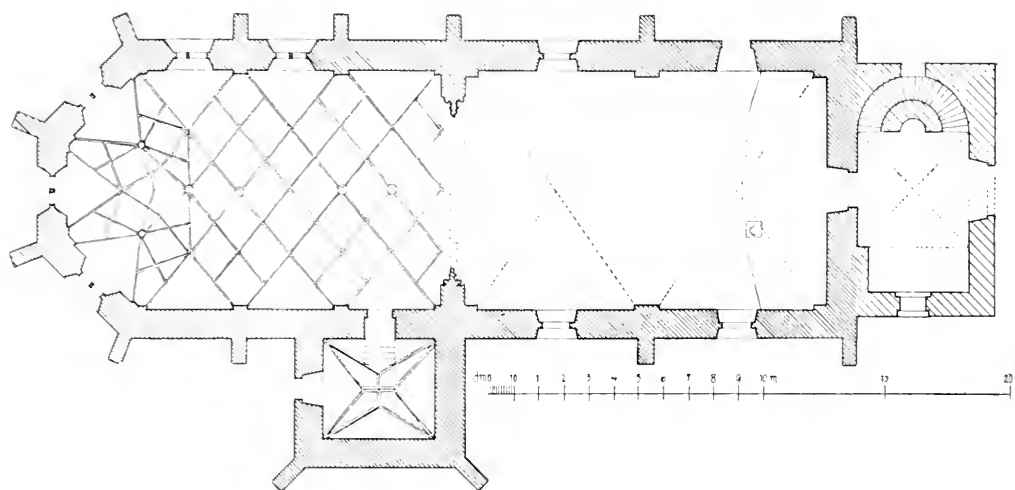
Obr. 227. Všeruby. Kostel sv. Ducha, Pádorys.
