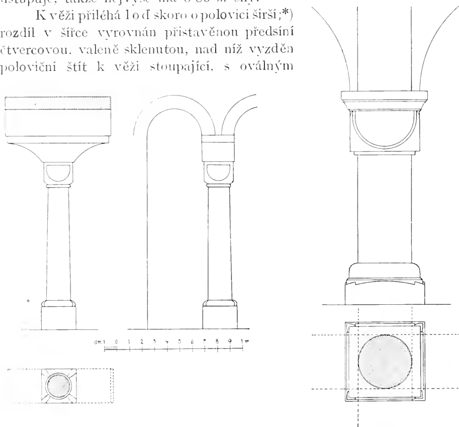
Obr. 199.—200. Svojsín, Kostel sv. Petra a Pavla. Okenní sloupky v 2. patře věže a klenební sloup v přízemí.
