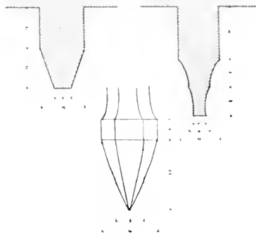
Obr. 102. Pernarec, Kostel sv. Mikuláše. Profil žebra klenby v sakristii a kněžišti a konsola.
