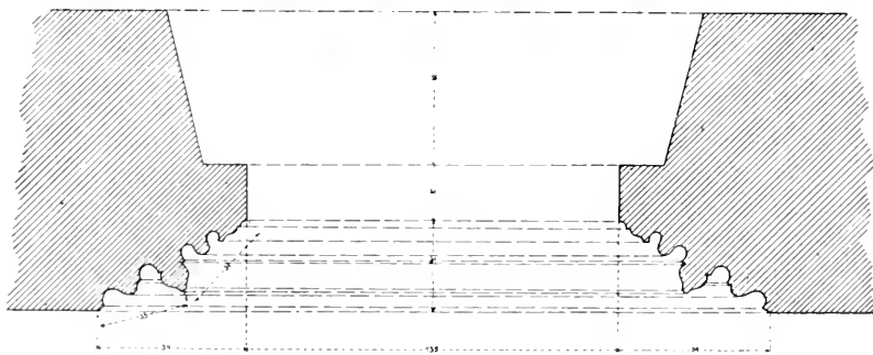
Obr. 172. Sulislav, Kostel sv. Vavřince. Portal do lodi a fez jeho ostění.
