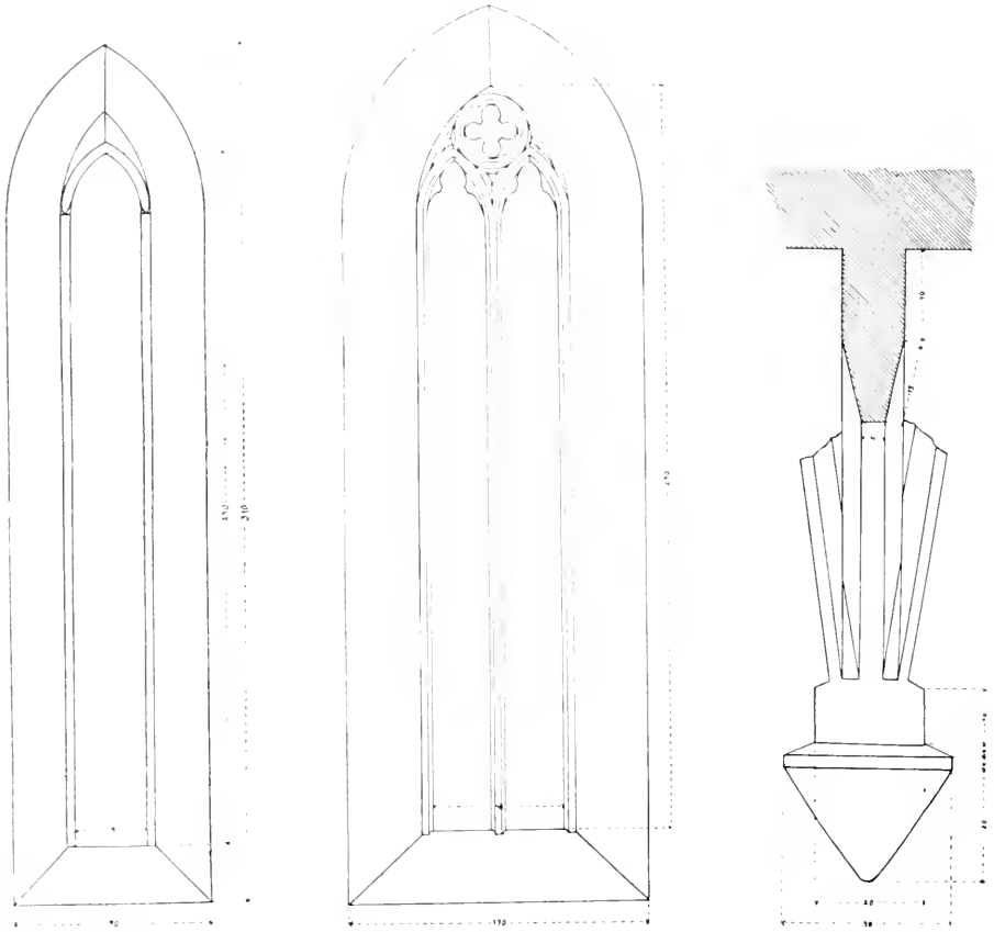
Obr. 107.—109. Prostibor. Kostel sv. Mikuláše. Okna a profil žebra a konsola klemby v kněžišti.
