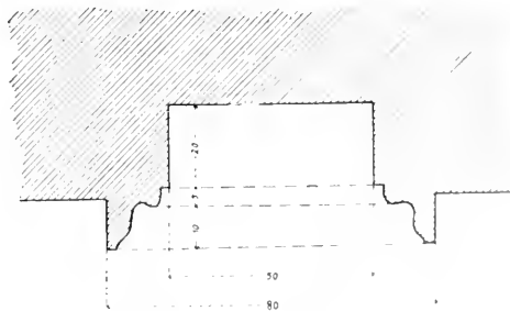
Obr. 90. Kostelec. Kostel sv. Jana Křtitele, Sanktuarium. Pohled a řez vyklenkem.
