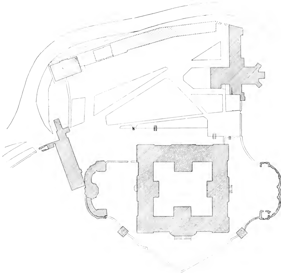
Obr. 46. Chotěšov, Klášter. Celková dispozice.
