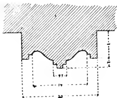
Obr. 70. Kladruby. Klášterní chrám P. Marie. Profily štukových žebor klenebních.
