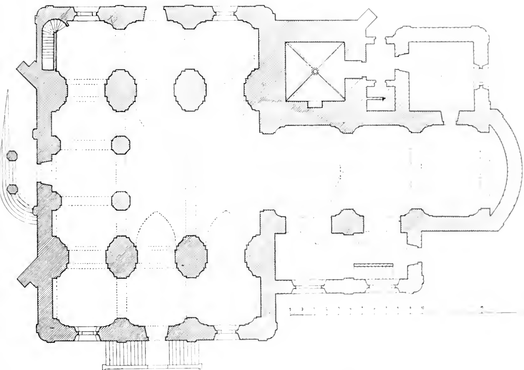
Obr. 134.—135. Stříbro. Kostel Vše ch Svatých. Řez podélný a pudorys.
