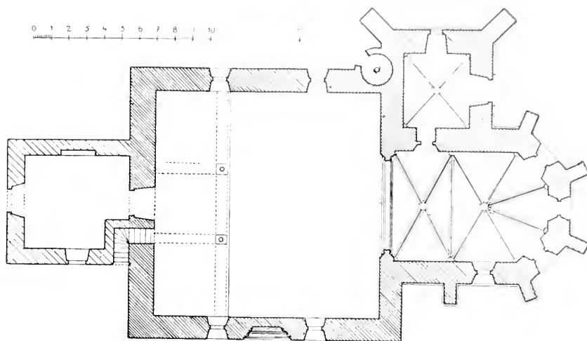
Obr. 86. Kostelec. Kostel sv. Jana Křtitele. Půdorys.
