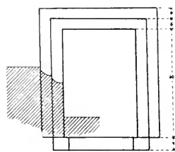
Obr. 131. Stříbro. Věž na mostě. Okénko (narys a řez ostěním).
