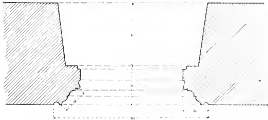
Obr. 196. Sulislav, Kostel sv. Vavřince, Portálek do sakristie a řez jeho ostěním.
