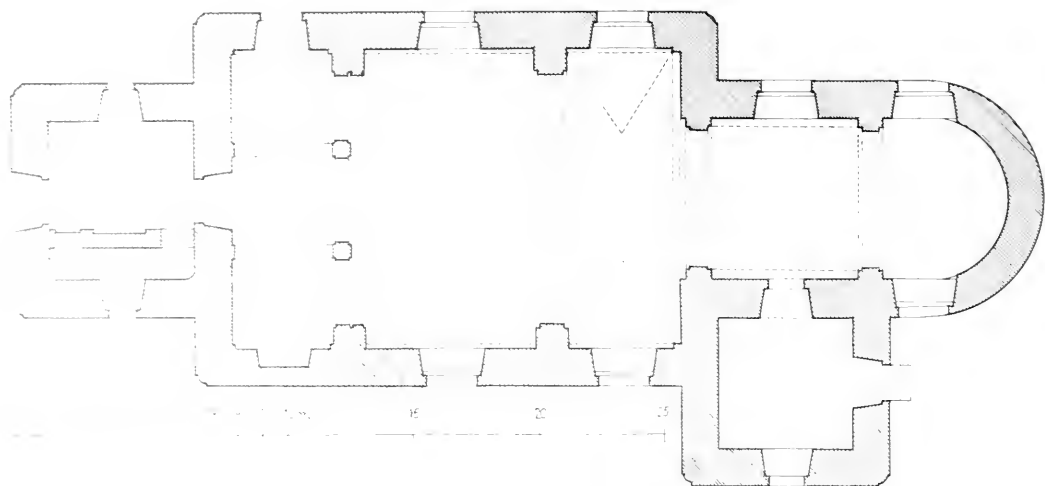
Obr. 59. Kladruby, Kostel sv. Jakuba, Pučorys.
