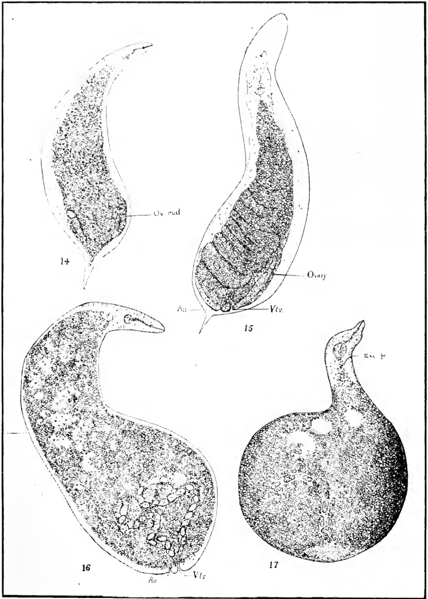
HETERODERA RADICICOLA.
