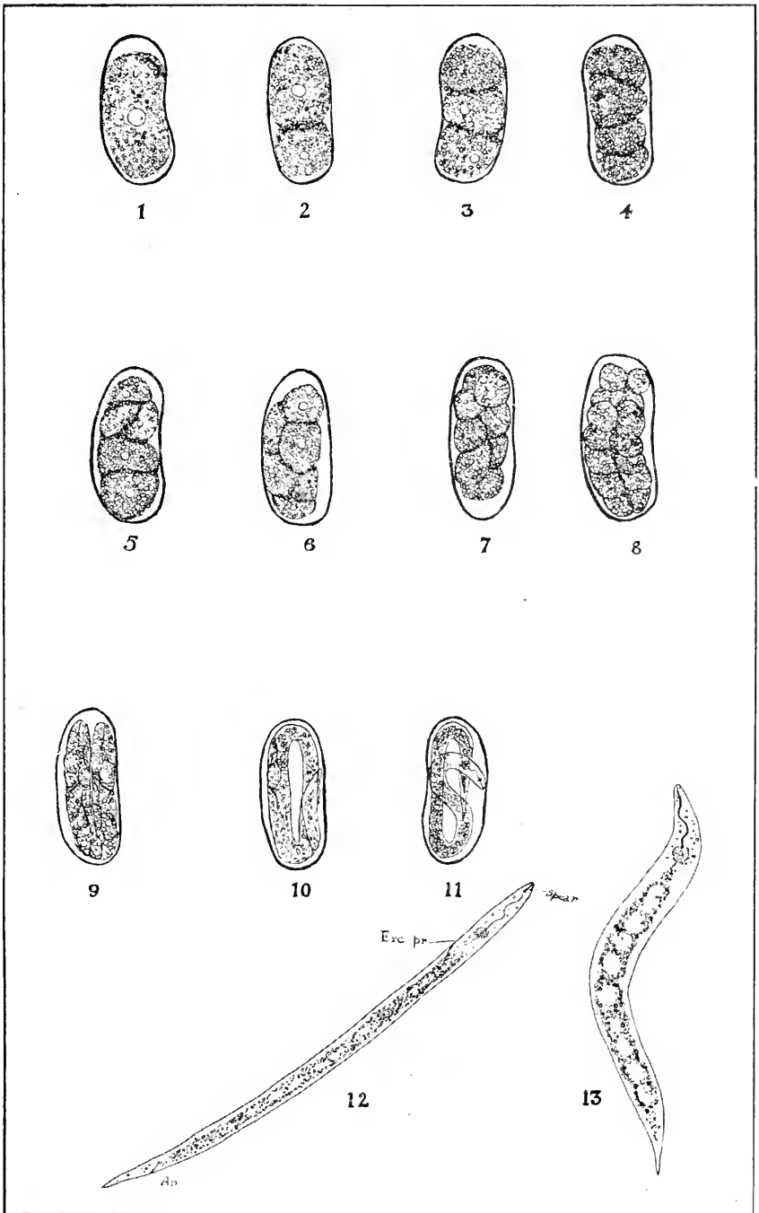
HETERODERA RADICICOLA.
