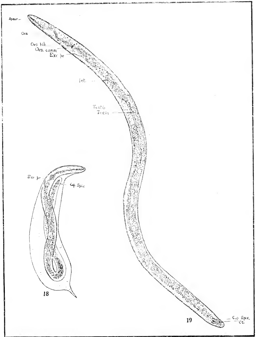
HETERODERA RADICICOLA.
