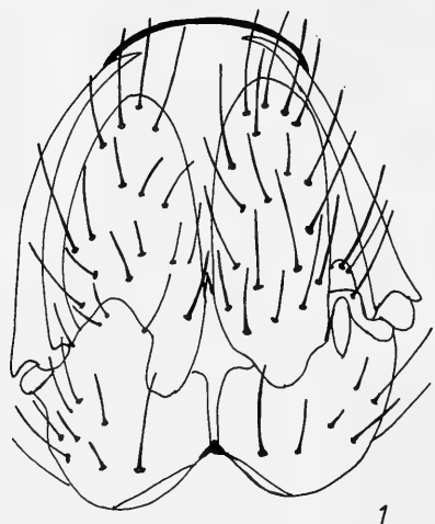
Abb. 1: Boletina abdita sp. n. Hypopygium dorsal.
