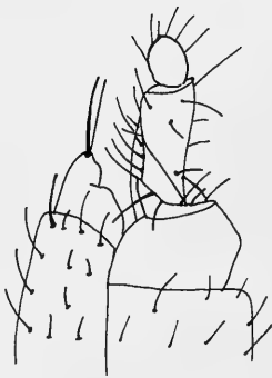
Abb. 3: Boletina abdita sp. n. Legeröhre lateral.
