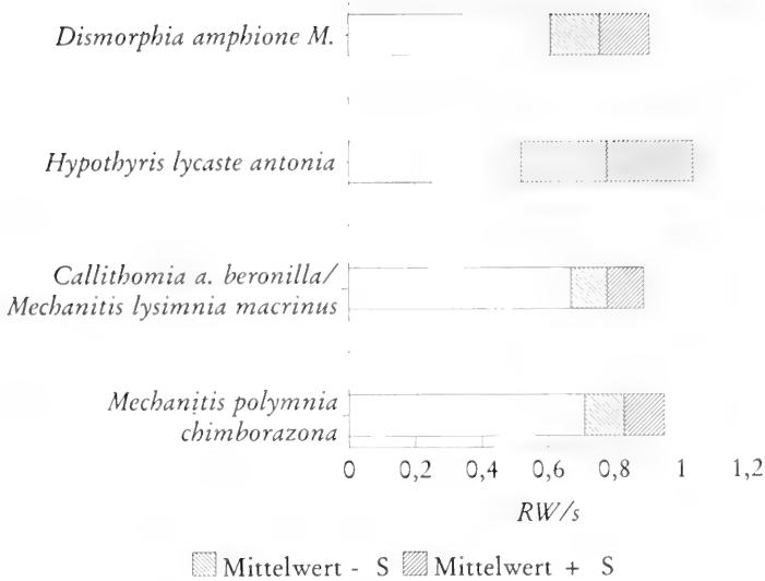
Abb. 4.12. Mittlere Häufigkeiten der Flugrichtungsänderung pro Sekunde (RW/s) von Dismorphia amphione und einigen ihrer Vorbilder (15 km bzw. 17 km östlich von Sto. Domingo de los Colorados, 700 m über NN).
