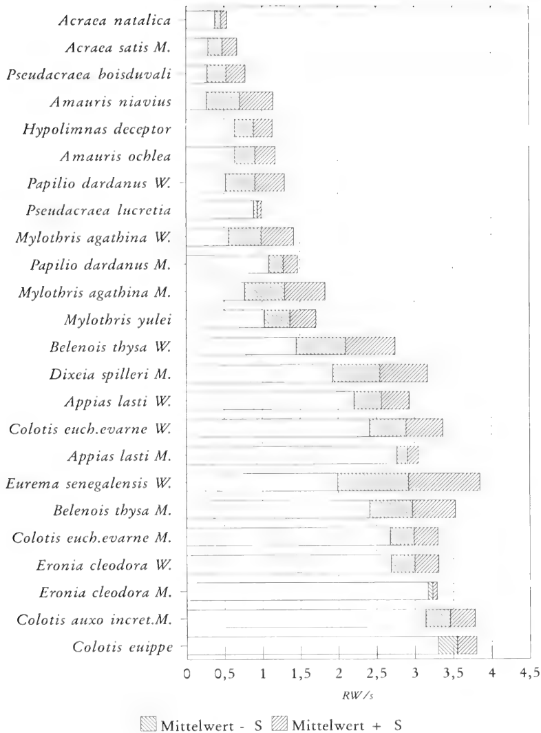
Abb. 4.2. Durchschnittliche Häufigkeit des Flugrichtungswechsels pro Sekunde einiger, soweit feststellbar, nicht erschreckter bzw. balzender Falterarten Kenias . RW/s: Mittelwert der Richtungswechsel pro Sekunde. S: zugehörige Standardabweichung.
