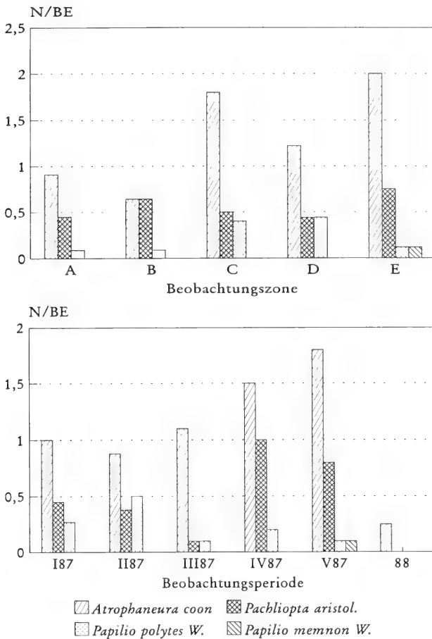
Abb. 4.4. Örtliche und zeitliche Häufigkeitsverteilung der Papilioniden Atrophaneura coon , Pachliopta aristolochiae und der mimetischen Weibchen von Papilio polytes und Papilio memnon im Khao Phra Thae-W-Park auf Phuket (Thailand). (Erklärung der Zonen A-E bzw. der Zeitperioden I87-V87, 88 vgl. Abb. 2.1 bzw. Tab. 3.1-3.)
