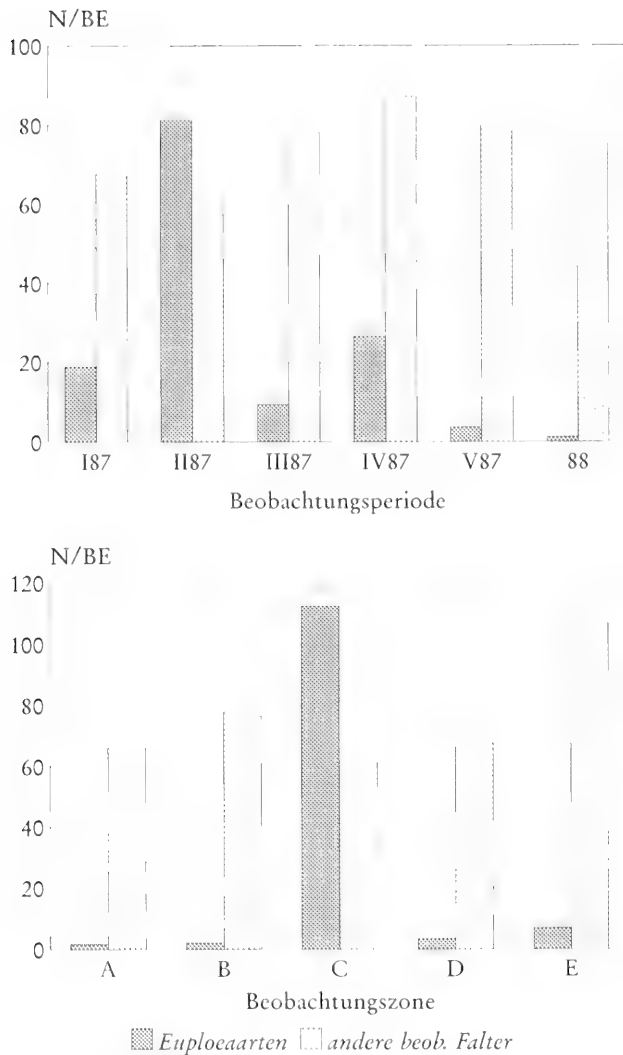
Abb. 4.8. Zeitliche und örtliche Häufigkeitsverteilungen der Euploea -arten im Vergleich zu den übrigen tagfliegenden Schmetterlingen im Khao Phra Thaew-Park auf Phuket (Thailand). (Zahlenwerte: vgl. Tab. 4.9, S. 47)
