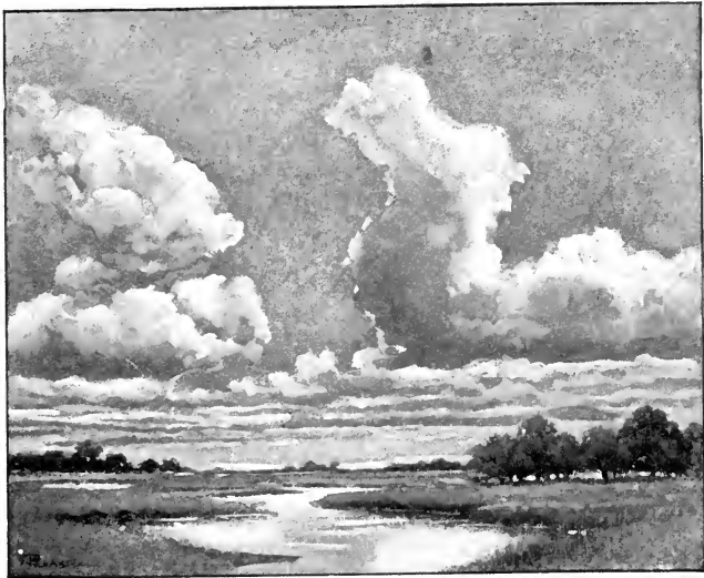
CUMULUS CLOUDS
