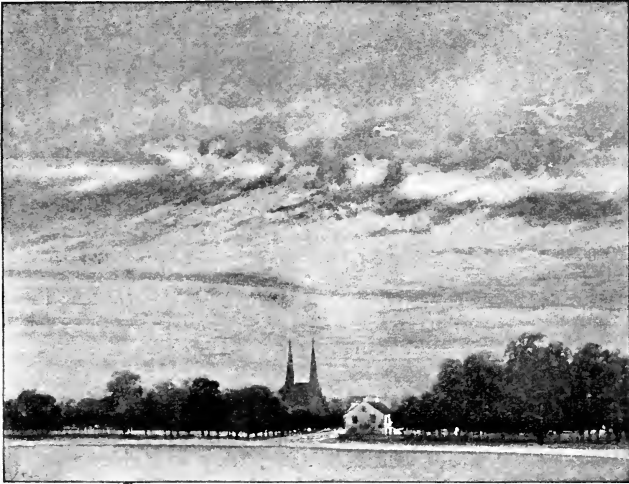
CIRRUS CLOUDS
