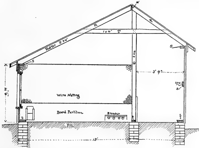
FIG. 2—HAMMONTON BROODING HOUSE
