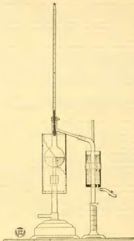
FIG. 6.—Distillation apparatus.
