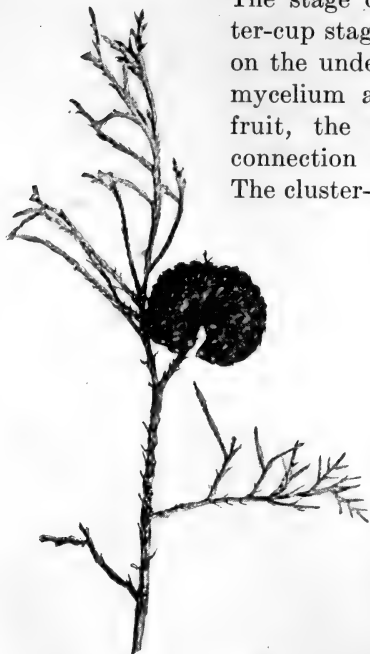
FIG. 144.—A cedar-apple.
