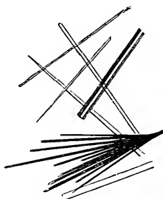
FIG. 18. SODIUM GLYKOCHOLATE.
