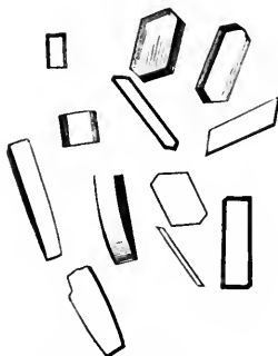
FIG. 21. GLYCOCINE.
