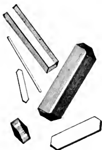
FIG. 19. CHOLALIC ACID.
