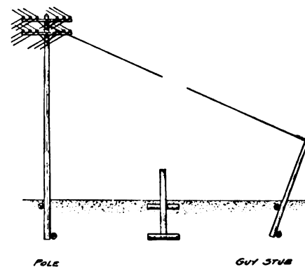
FIG. 2.—CRIB BRACING
