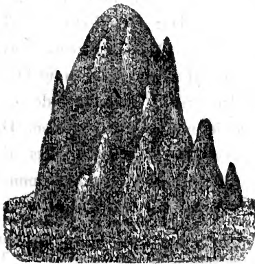
En Termithei, opført af Termes bellicosus (efter Smeathman).
