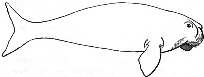
Omrids af den nulevende Dygong for at give en Forestilling om Dinotheriets Legemsform, der uidentvilt har været den samme, men med den ovenfor afbildede Form af Hovedet.
