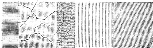
Havet. Vaddene. Forlandet. Marsken. Gesten. (med Vadstrømmene).
