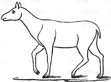
Omrids af det slanke Anoplotherium. ( Anoplotherium gracile ).
