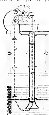
Ketjupumppu.
