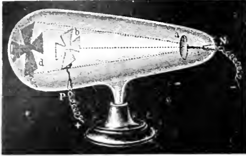
Crookesin putki.
