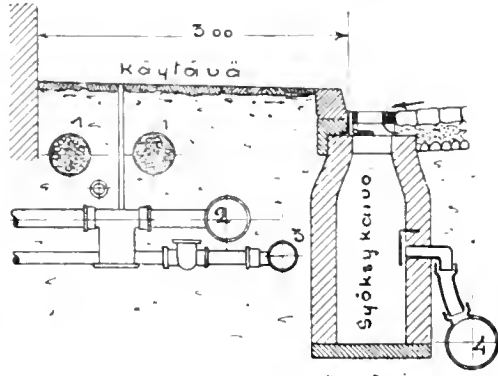
1. Sähköjohtotortvia. 2. Kaasujohto. 3. Vesijohto. 4. Likaviemäri.
