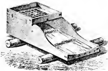
Huuhtomaränni.
