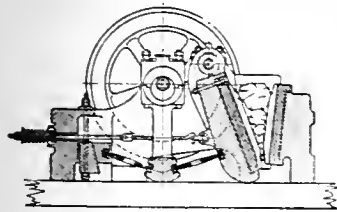
Kivenmurskaaja.
