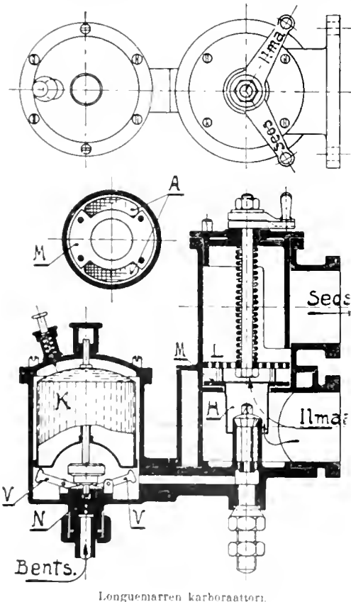
Longuemarren karboraaattori.
