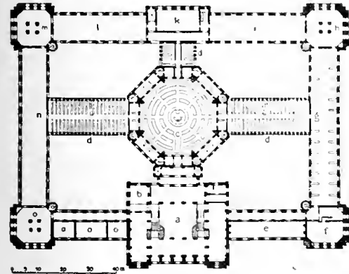
Washingtonin kongressikirjaston pohjapiirros.
