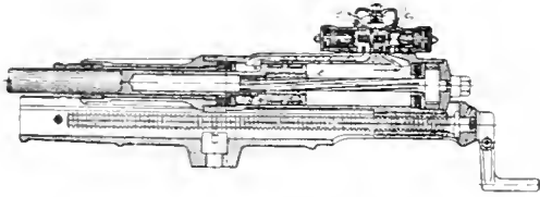
Kuva 3. Painelmaporakone.
