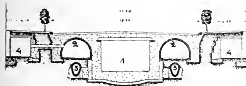
1. Rautatietunneli. 2. Tunneli erilaisia johtoja varten. 3. Likajohtotunneli. 4. Rakennuksen kellari.
