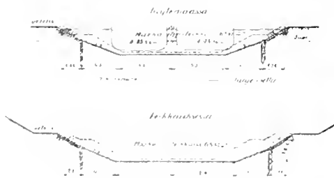
Kuva 1. Saimaan kanavan säännöllinen poikkileikkaus Mustolan ja Sujanamaarven välisellä osalla
