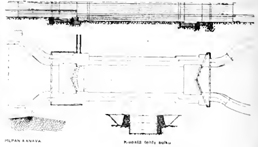
Kuva 2. Sulun pohja- ja leikkauksuvia.
