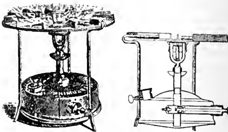
Primus-keittiö.
