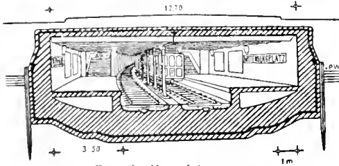
Kuva 3. Maanalainen rata.
