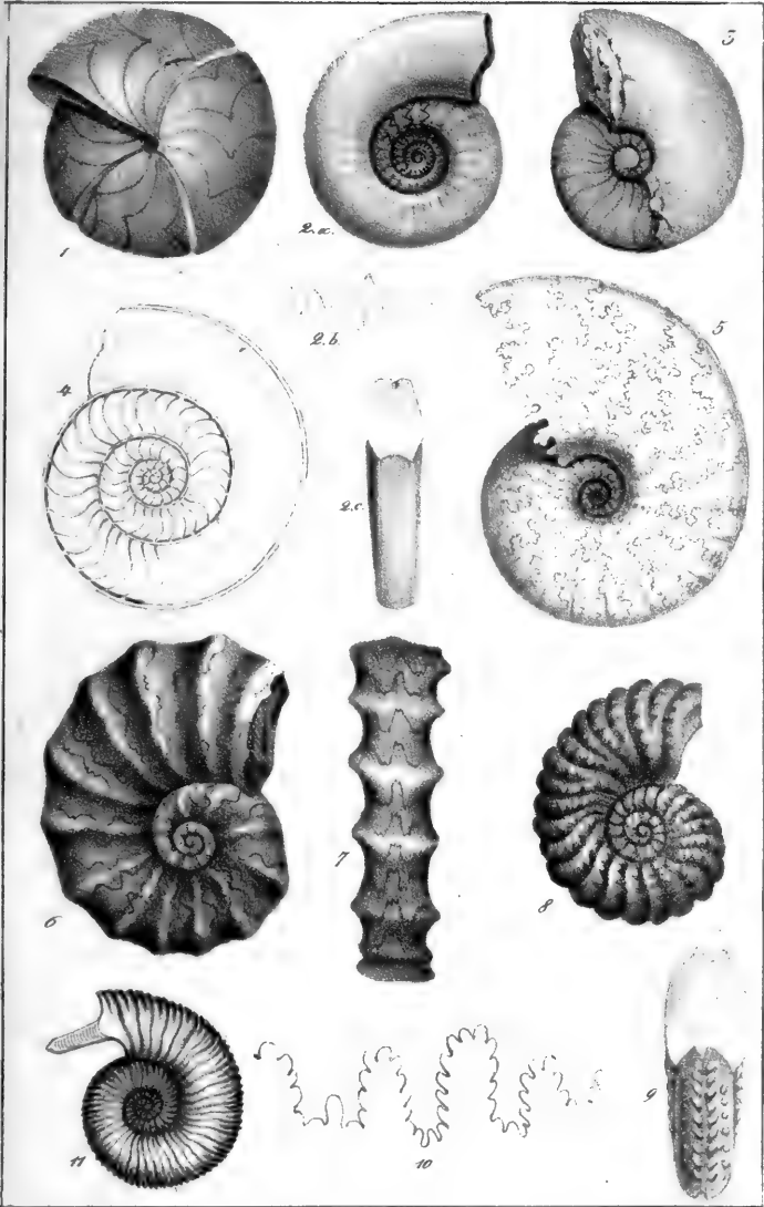
1 - 3 Goniatites 4 - 11 Ammonites.
