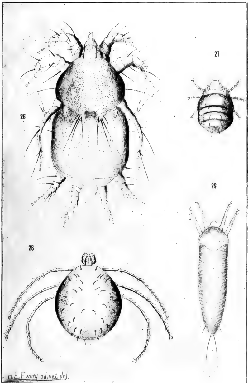
TRUE PARASITES.
