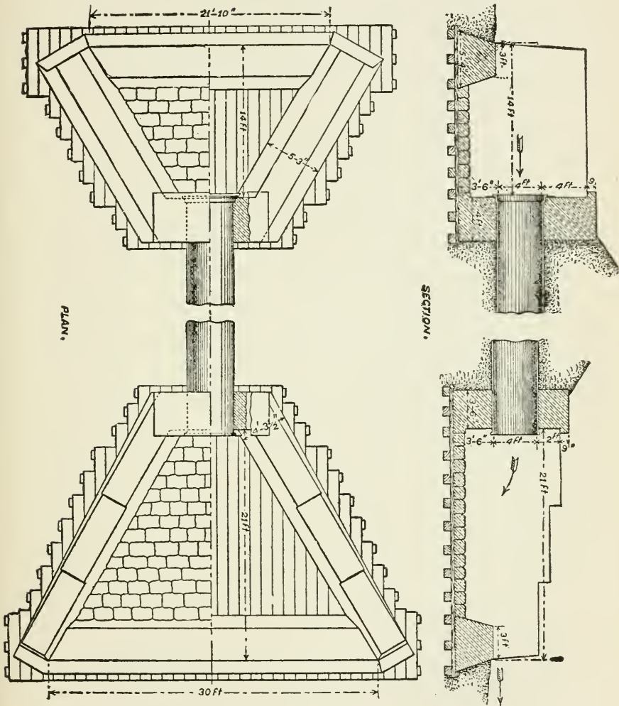
FIG. 101.—CAST-IRON PIPE CULVERT.—C., B. & Q. R. R.
