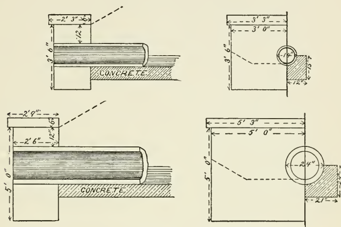
FIG. 99.—STANDARD VITRIFIED PIPE CULVERT.—K. C. &amp; O. R. R.
