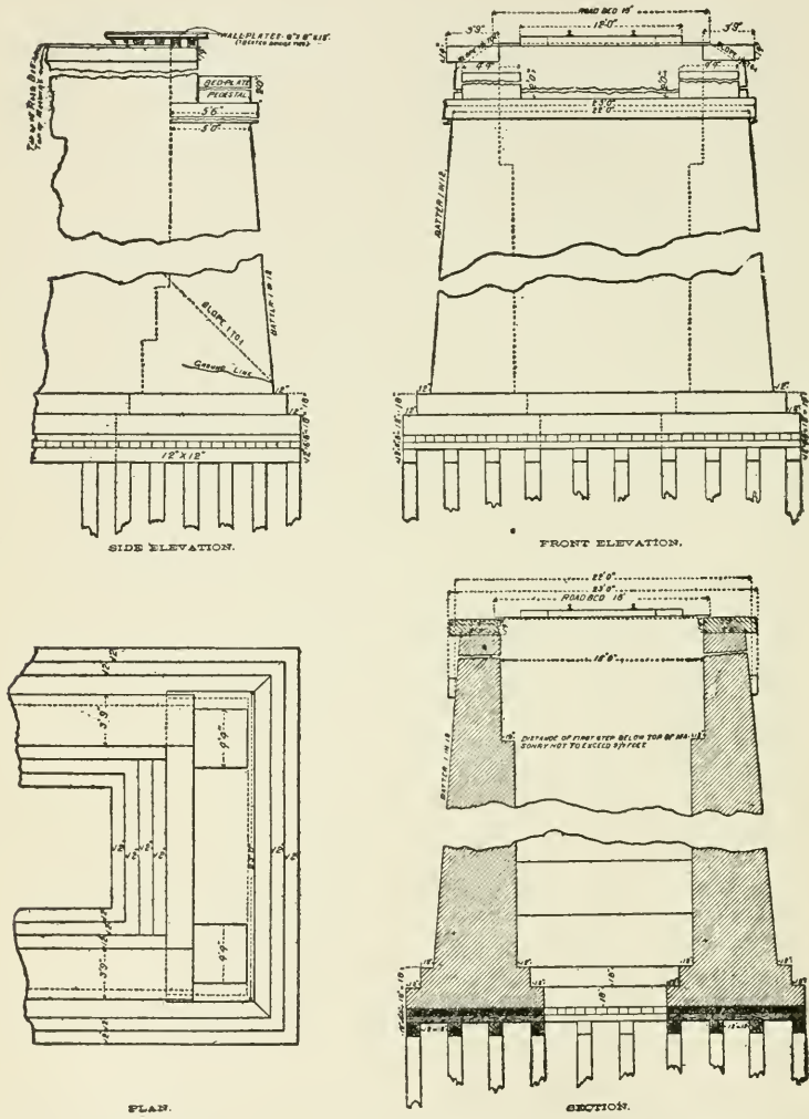
FIG. 83.—U ABUTMENT.—A. T. & S. F. R. R
