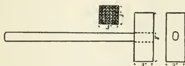
FIG. 15.—BUSH HAMMER.
