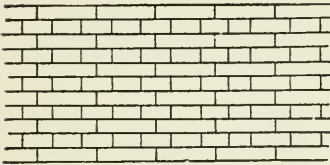
FIG. 48.—ENGLISH BOND.
