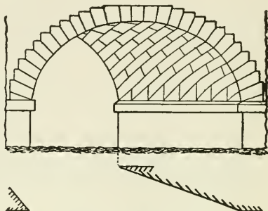
FIG. 112.—SKEW ARCH.
