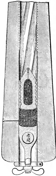
FIG. 367 and 368.—The Währendorf breech-loader.
