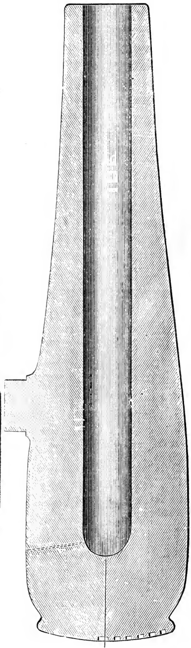
U. S. HOLLOW-CAST COLUMBIAD.
