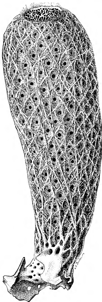
FIG. 18. Regadrella phoenix , O.S. (After Agassiz.) \frac{3}{4} .
