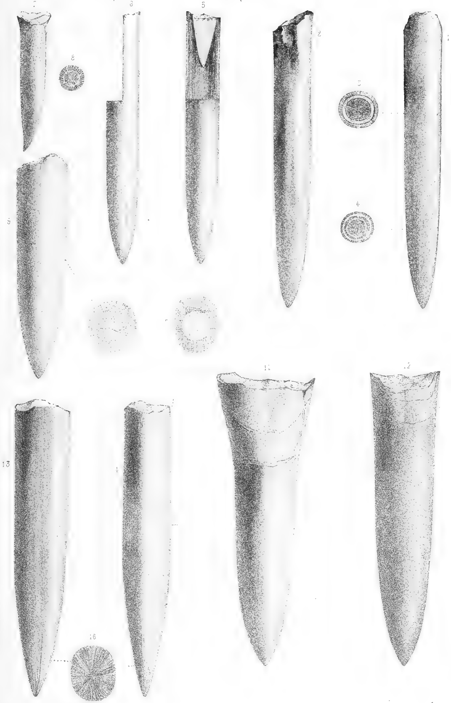
Ammonites Jurassiques.
