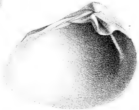
Trilobites ? Murchisonia
