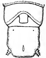
Fig. 9. Chl. Strandii , ♂, von unten.
