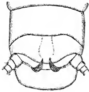
Fig. 8. Chl. Strandii , ♂, von oben.
