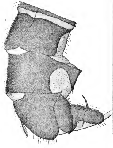
Fig. 5. Leuctra Rosinae ♂, von der Seite.
