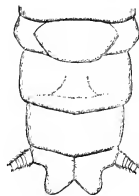
Fig. 4. Isogenus Nanseni , ♀, von unten.
