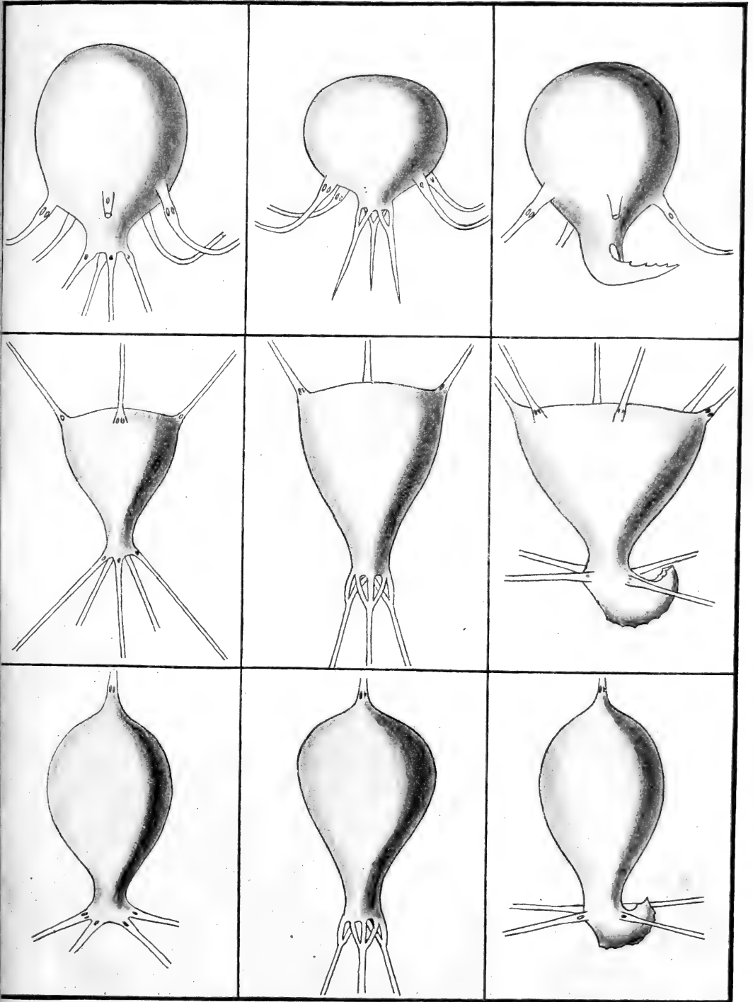
Fig. 8. Neun Tuscaroridae, die verschiedenen Kombinationen der drei Peristomtypen und der drei Hauptstellungen der Radialstacheln darstellend (siehe Tabelle). 1, 2, 3 Vertikalreihe: kelchförmiger, korbformiger, helm- oder schnabelförmiger Peristomtypus; 1, 2, 3 Horizontalreihe: circoreale, aborale, apicale Stachelstellung.
