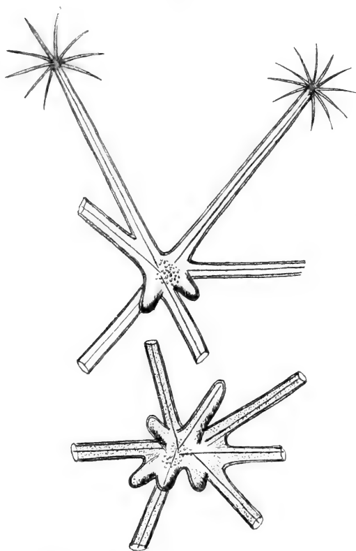
Fig. 5. Knotenpunkte aus einem unfertigen Skelet von Sagenoarium anthophorum n. sp. Die sekundäre Füllsubstanz beginnt erst sich abzuscheiden, die Primitivnadeln sind noch deutlich zu erkennen. ( Sagenoarium anthophorum n. sp. Gipfelstacheln mit einer palmenähnlichen Krone von 6—12 Terminalästen, daneben vielfach kürzere Gipfelstacheln mit 2—4 kurzen, horizontal abstehenden Haken. Fundort: T.St. 135, Schl.N. 680—480, Antarcis.)
