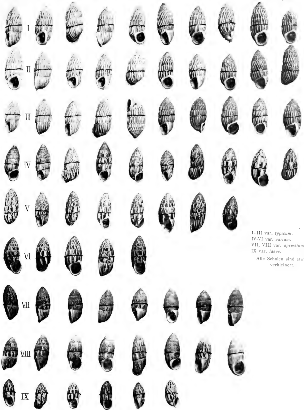
Formenkette von Cerion glans KÜSTER in der Richtung von West nach Ost auf New Providence (I-VIII) und Eleuthera (IX).
