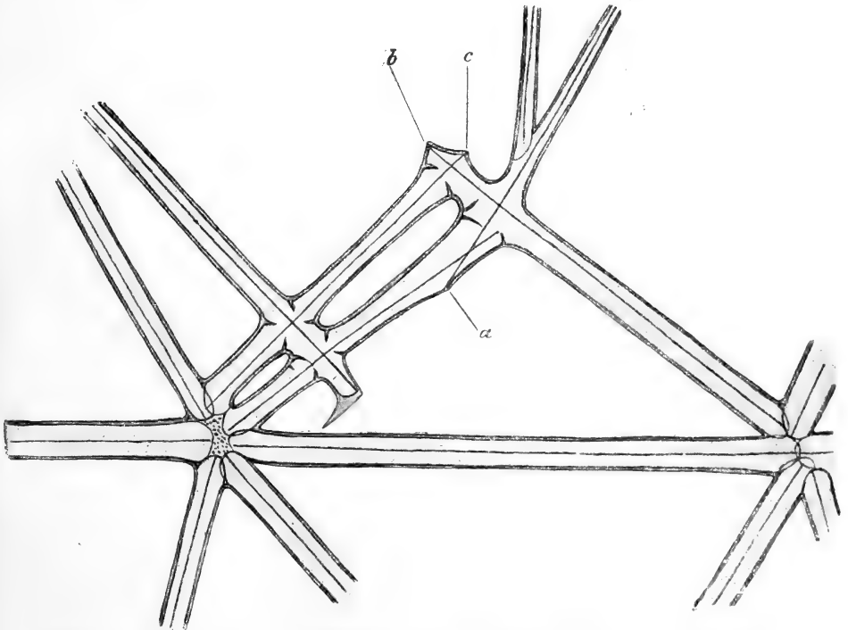
Fig. 4. Partie aus einem monströsen Aulosceca -Skelet. Bei a, b, c Vorstülpungen der primären Kiesellamelle, durch die vorspringenden Enden der Primitivnadeln hervorgerufen.
