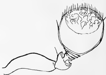
Fig. 4. Xyleborus excavatus Hagedorn. Linker Fühler. Vergr. 223/1.
