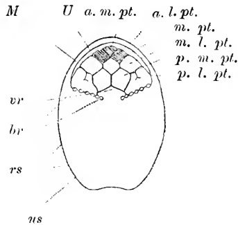
Figur 2. Tremataspis Schmidt , Rohon. Obersilur von Oesel in Russland. Untere Flächenansicht des Kopfes, teilweise reconstruirt. 21) U = Umschlagsrand des oberen Kopfschildes, ns = unteres Kopfschild, M = Mundspalte, br = Kiemenöffnungen, vr = mittlerer Vorsprung des unteren Kopfschildes, a. m. pt. = vordere Mittelplatte, a. l. pt. = vordere Seitenplatte, m. pt. = mittlere Platte, m. l. pt. = mittlere Seitenplatte, p. m. pt. = hintere Mittelplatte, p. l. pt. = hintere Seitenplatte. Natürliche Grösse.
