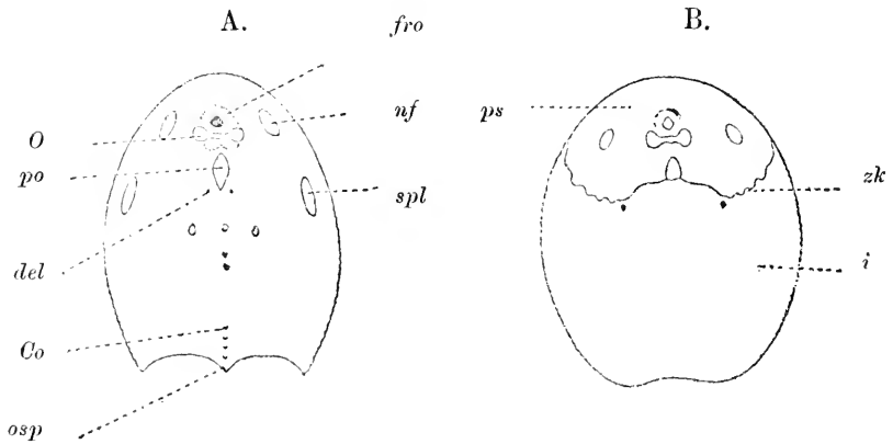
Figur 7 A, B. Tremataspis Schmidtii , J. V. Rohon. Obersilur der Insel Oesel in Russland. A = Oberes Kopfschild, B = Unteres Kopfschild. 29) fro = Frontalorgan, nf = Nasenöffnung (?), spl = Spritzloch, po = Parietalorgan, del = Ductus endolymphaticus (?), Co = Crista occipitalis , osp = Occipitalvorsprung, O = Aug nöffnung, i = unteres Kopfschild, zk = Zacken am Vorderrande des unteren Kopfschildes. Auerthalbmäßige Vergrößerung.
