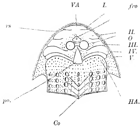
Figur 1. Thyestes verrucosus , Eichwald . Obersilur von der Insel Oesel in Russland. Obere Flächenansicht des Kopfes. Schematische Abbildung des oberen Kopfschildes und des Primordialcranium. Letzteres mit schärferen Linien unterhalb des Schildes eingezeichnet. VA = Vorderer Abschnitt des Primordialcranium, HA = Hinterer Abschnitt des Primordialcranium, rs = Randtuberkel des Schildes, Co = Crista occipitalis des Schildes, I, II, III, IV, V = die fünf Segmente des Primordialcranium, fro = Frontalorgan, O = Augenöffnung, po = Parietalorgan. Anderthalbmalige Vergrößerung.
