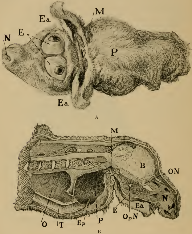
FIG. 30. CYCLOPS. LAMB.
