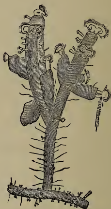
FIG. 5.— Limnias ceratophylli .
