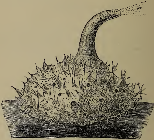
FIG. 24.— Spongilla fluviatilis .
