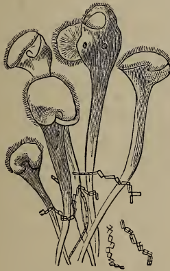
FIG. 10.— Stentor s.
