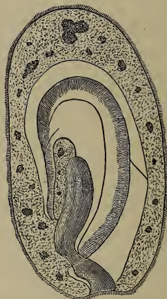
FIG. 11.— Bursaria truncatella .
