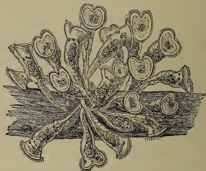
FIG. 23.— Megalotrocha ( albo-flavicans ).
