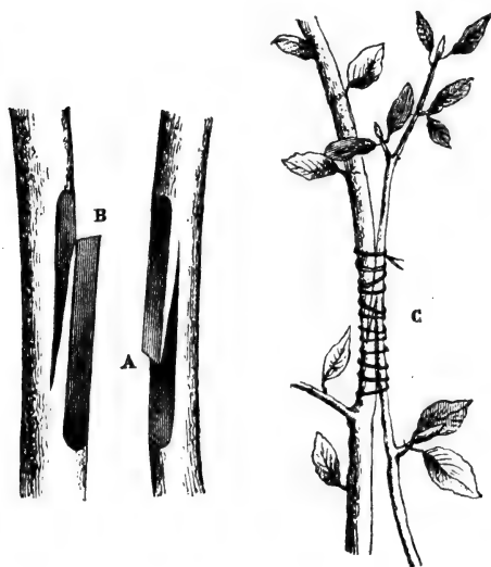
Сл. 51. Приљубљивање на лионски начин.
