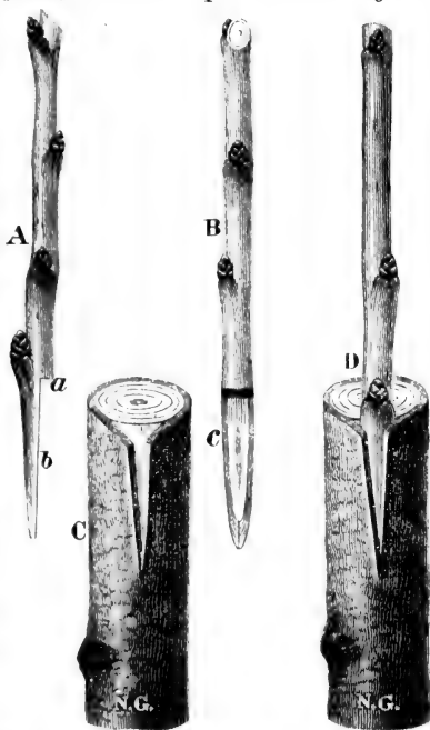
Сл. 74. АВ вијоке посматране спреда и по зади; С подлога с расцепљеном и одлубљеном кором; D изглед присада.
