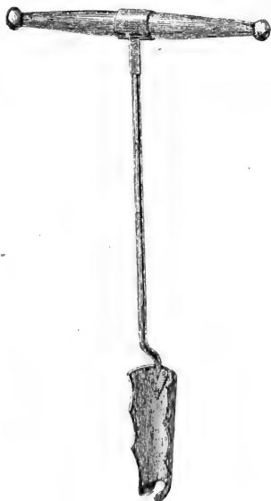
Сл. 192. Винцов сврдао за камените земље ( 1\frac{1}{10} природне величине).
