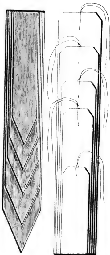
Сл. 118. Дашчице за обележавање сората, које се побијају у земљу испред вођака.
