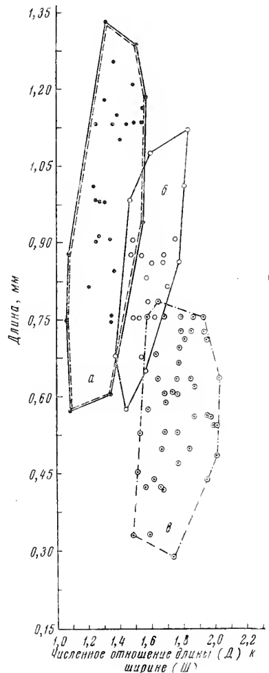
Рис. 6. Диаграмма рассеивания, показывающая зависимость между длиной раковин и степенью удлиненности
