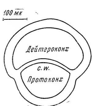
Рис. 1. Горизонтальное сечение нуклеококха (нефролепидинового типа) Lepidocyclus (рисунок сделан с помощью рисовального аппарата)
