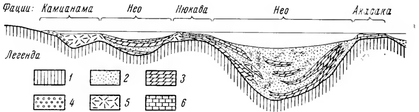
Рис. 4. Схематический фациальный профиль
