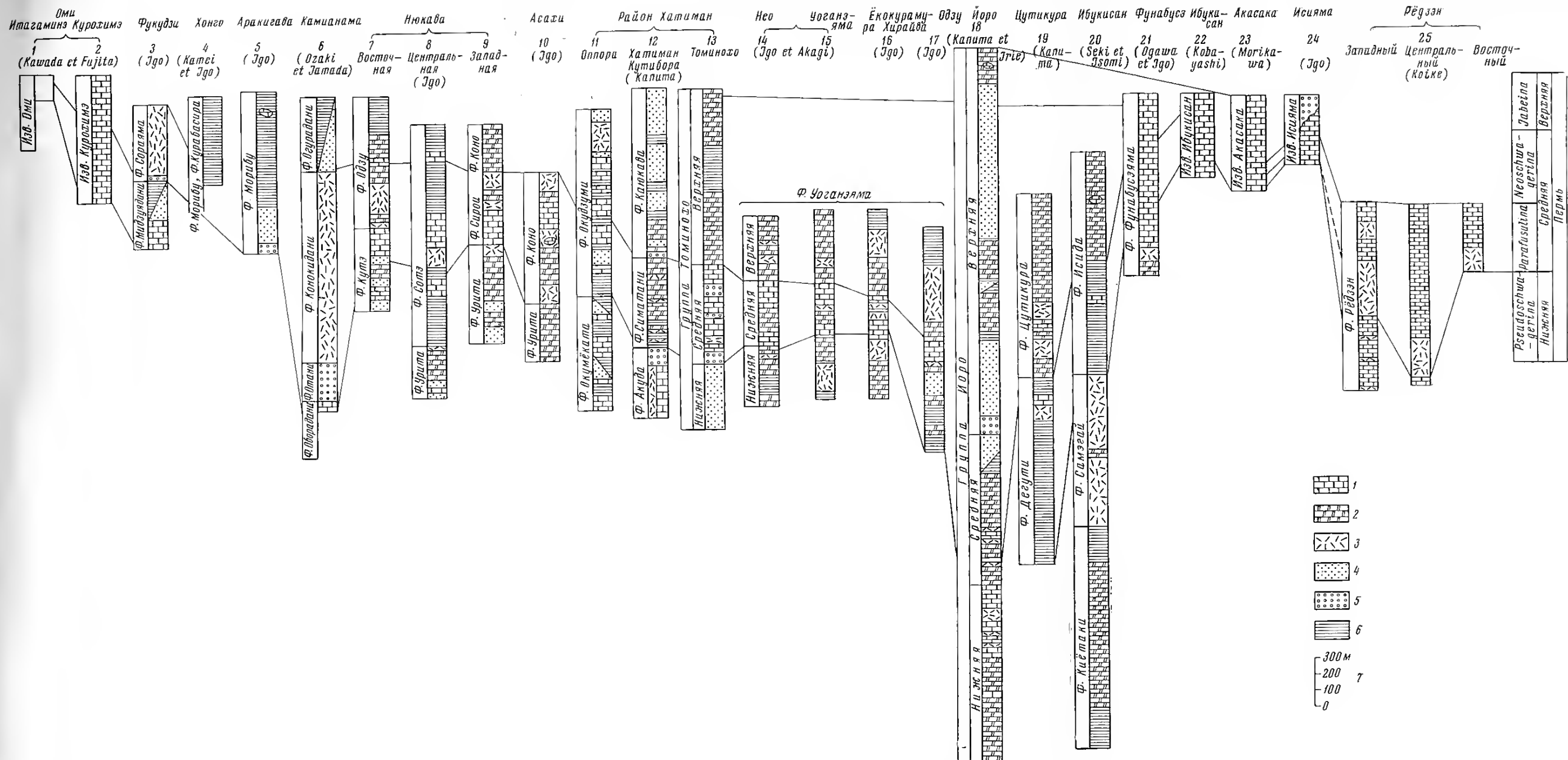
Рис. 1. Сопоставление разрезов пермских отложений массива Хиды
