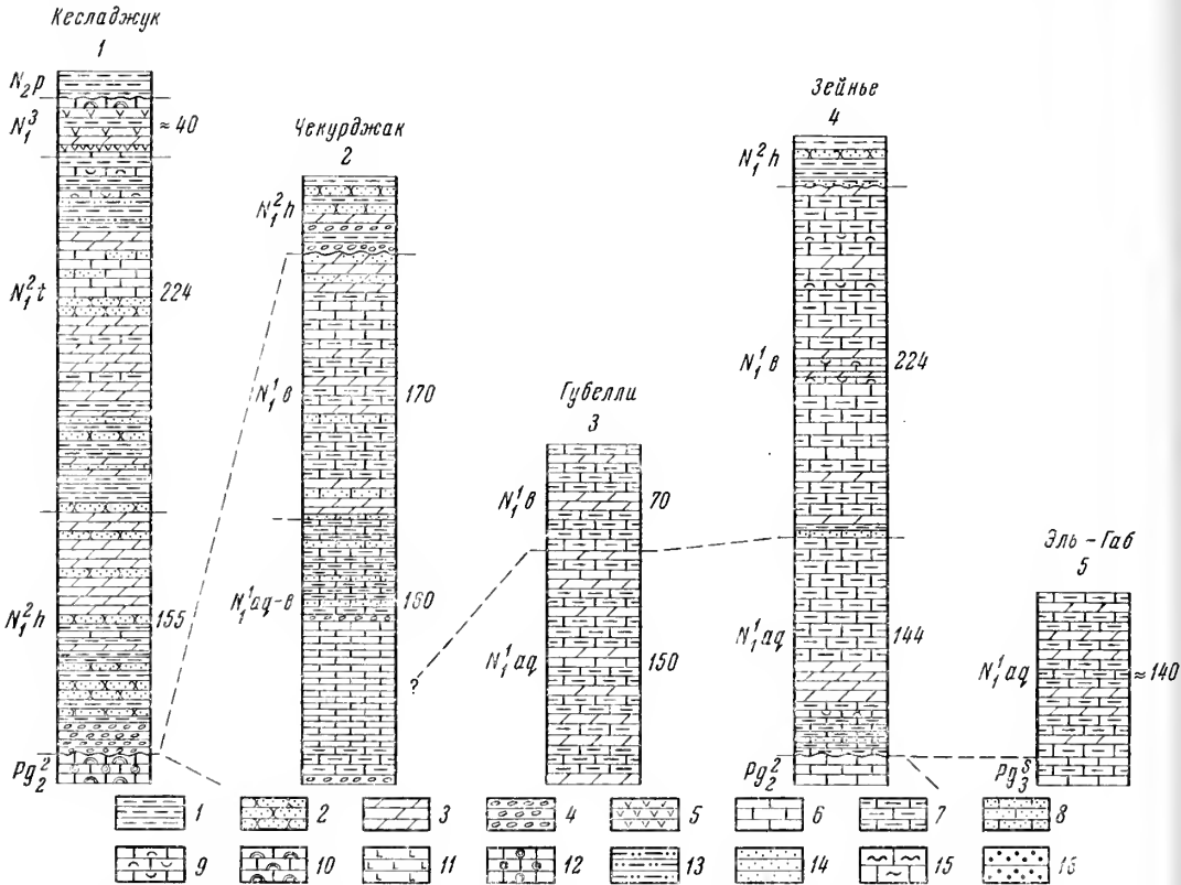
Рис. 2. Разрезы миоценовых отложений района Латакия и западной части впадины Эль-Габ 1 — глины; 2 — песчаники; 3 — мергели; 4 — конгломераты; 5 — гипсы; 6 — известняки; 7 — глинистые известняки; 8 — песчаные известняки; 9 — известняки-ракушечники; 10 — водорослевые известняки; 11 — эффузивные породы; 12 — нуммулитовые известняки; 13 — алевролиты; 14 — пески; 15 — окремненные известняки; 16 — гравелиты
