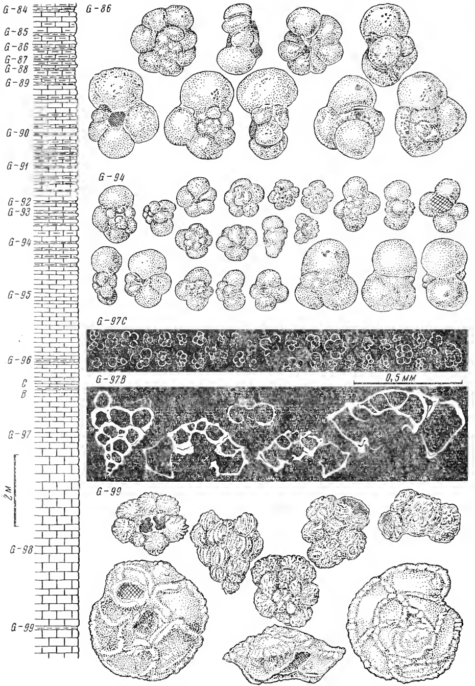
Рис. 1. Планктонные фораминиферы из пограничных между мелом и палеогеном отложений Центральных Апеннин (из Premoli Silva, Luterbacher, 1964)
