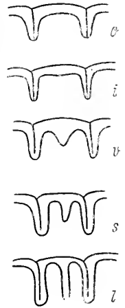
Рис. 2. Различные типы аксиальных септул
