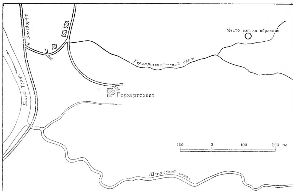
Рис. 2. План расположения мест взятия образцов в Герхартсрейтском овраге у Зигсдорфа
