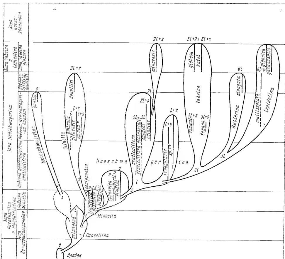
Рис. 4. Схема филогенетического развития подсемейства Neoschwagerinae и основные бносерии, а также типы аксиальных септул у важнейших видов
