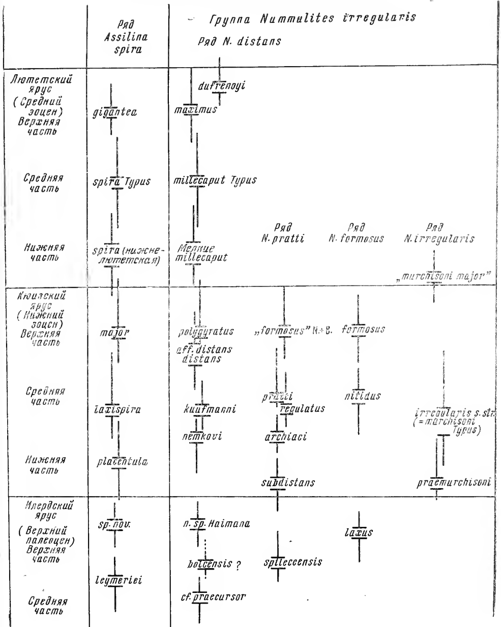
Филогенетические соотношения в пределах ряда Assilina spira и рядов группы Nummulites irregularis
