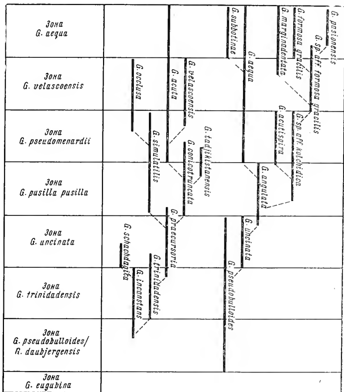
Рис. 3. Стратиграфическое распространение некоторых глобороталиид в Центральных Апеннингах и их предполагаемые филогенетические связи
