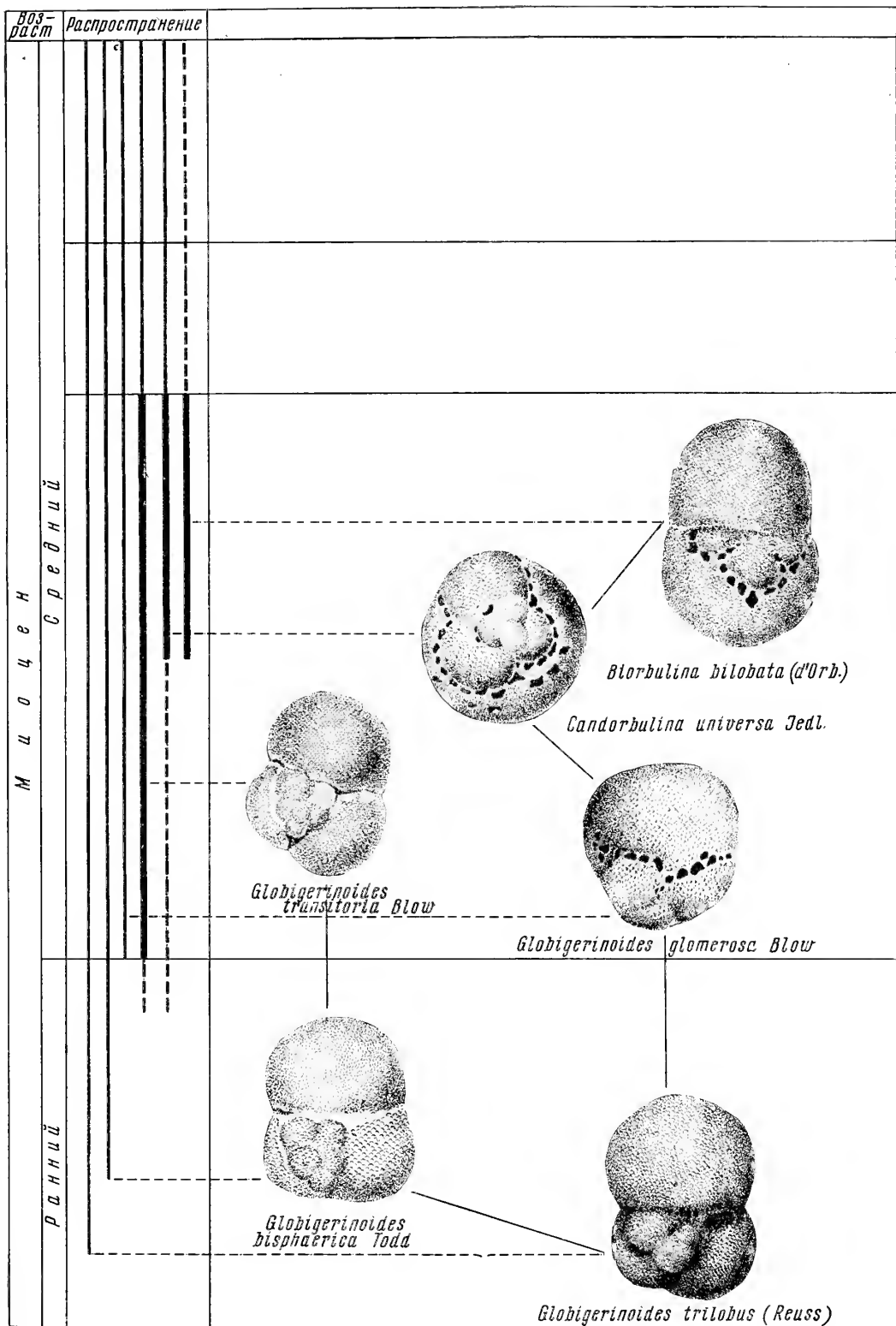
Рис. 2. Схема генетических взаимоотношений родов Globigerinoides , Candorbulina , Biorbulina (рисунки выполнены художником Л. Ф. Цыськ)
