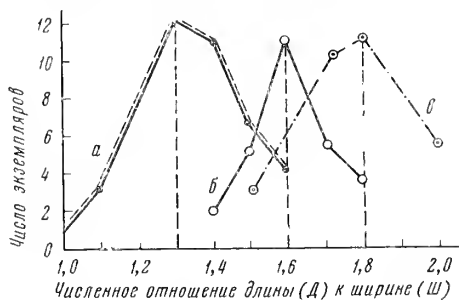
Рис. 4. Кривые изменения степени удлиненности раковин силикосигмолин
