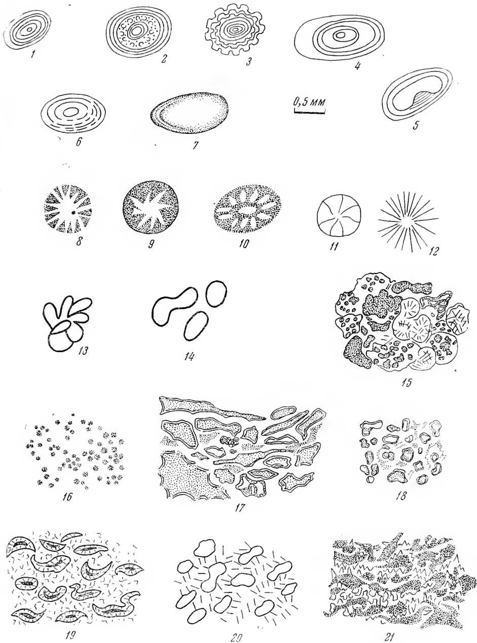
Рис. 2. Схемы строения различных групп микрофитолитов
