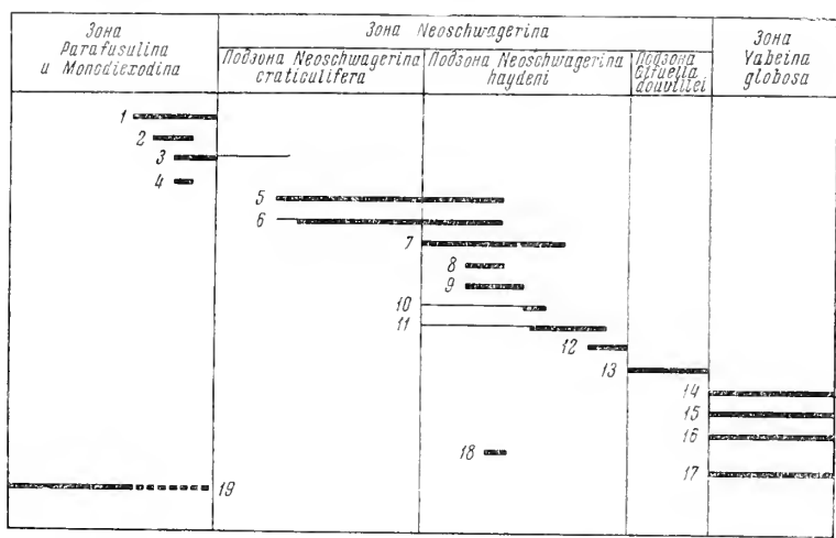
Рис. 5. Схема стратиграфического распространения важнейших неосвагеринид в Японии
