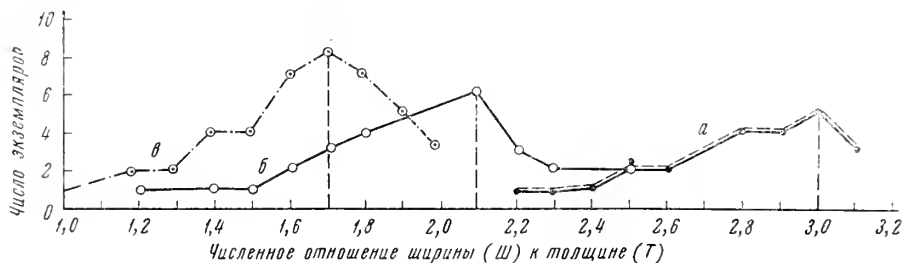
Рис. 5. Кривые изменения степени вздутости раковин силикосигмонид а — Silicosigmoilina sp.; б — S. californica Cushman. et Church.; в — S. perplexa Isr.
