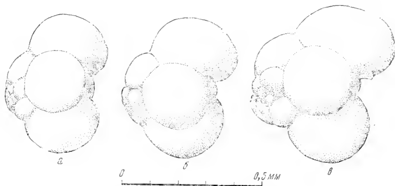
Рис. 4. Эволюционный ряд Globigerina eosaena Gumbel — G. corpulenta Subbotina — G. gortanii (Borsetti). Вид сбоку. Нижний олигоцен, Рейт-в-Винкле, Баварские Известняковые Альпы (образец 3056)
