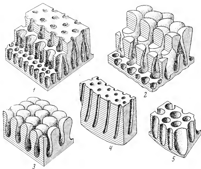
Рис. 2. Блок-диаграммы, иллюстрирующие строение стенки у некоторых представителей семейства Spirocyclinidae
