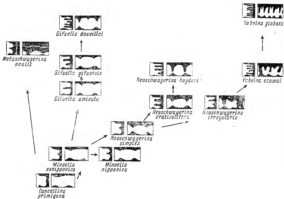
Рис. 1. Характер септул (по Нопжо, 1959) у видов подсемейства Neoschwagerinipinae. Для каждого вида на левой части рисунка изображены аксиальные септулы, на правой — поперечные септулы и в основании каждого рисунка — парахоматы; поперечные септулы второго порядка являются зачаточными или редкими у видов Minoella nipponica , Neoschwagerina craticulifera , N. haydeni , Gifuella amiculæ и G. gifuensis и не изображены
