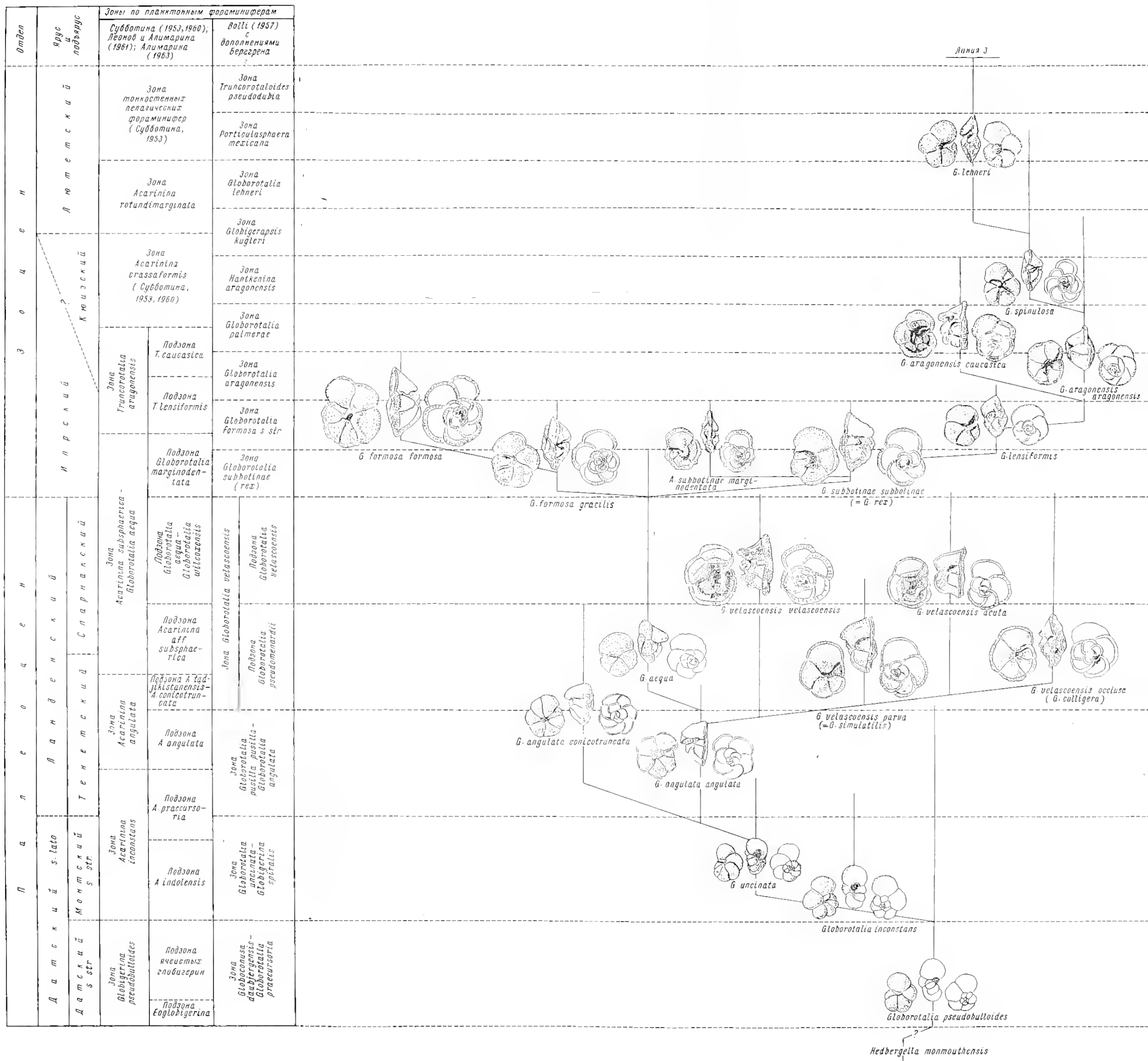
Рис. 2. Предполагаемое филогенетическое развитие палеогеновых кошеческих глобороталид
