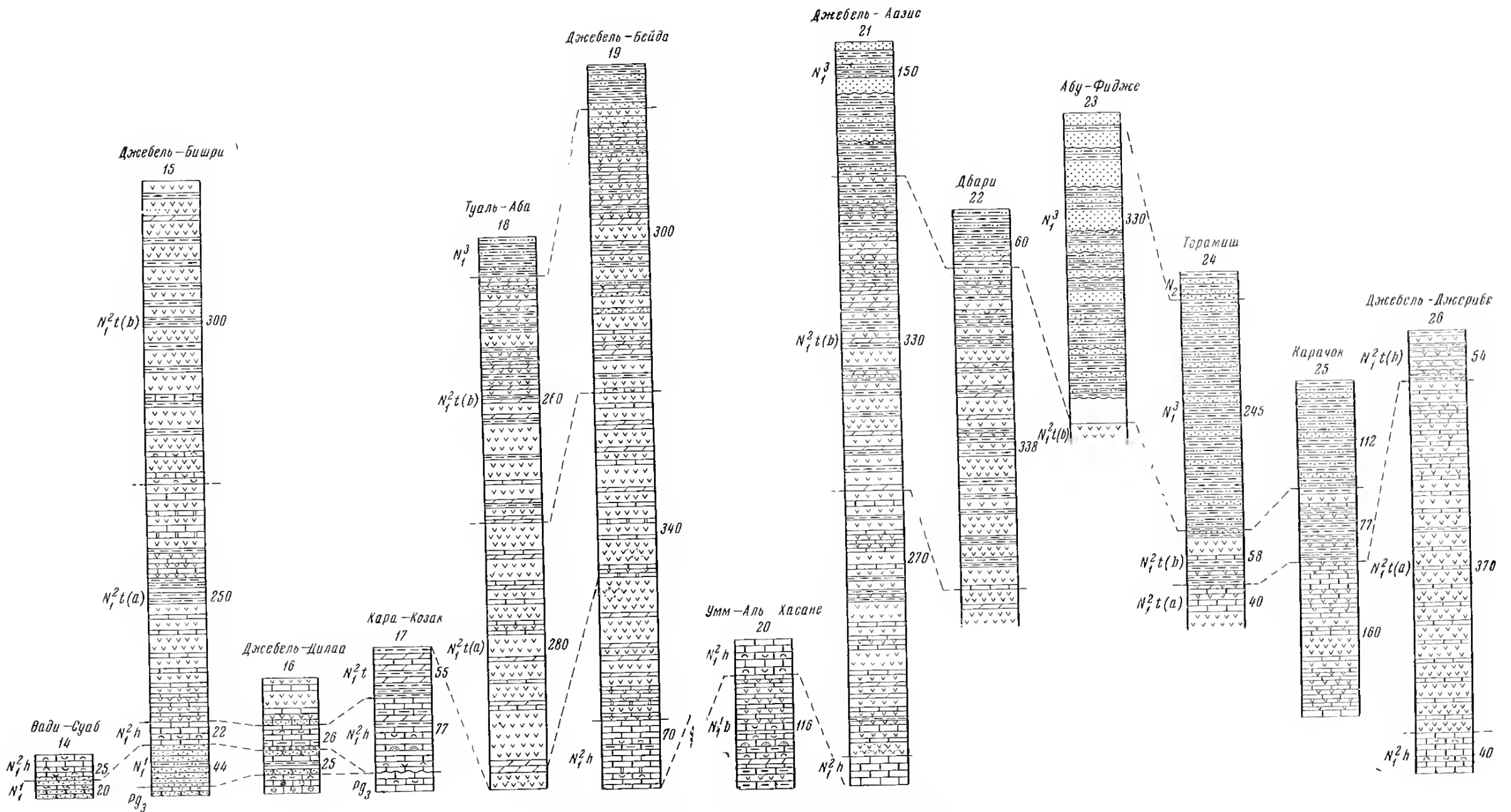
Рис. 4. Разрезы миоценовых отложений Месопотамской впадины Условные обозначения те же, что на рис. 2
