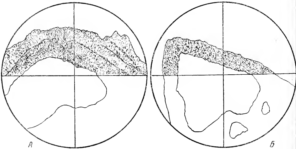
Фиг. 1. Схемы неясно радиально-лучистой микроструктуры стенки у Elphidium latusovum sp. nov. (А) и зернистой стенки у Canalifera eichwaldi (Bogd.) (Б). Николи скрещены, \times 800 .
