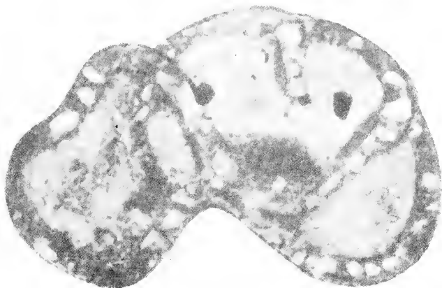
Фиг. 2. Endothyranopsis ex. gr. crassus (Brady). Скошенное поперечное сечение. В стенке раковины хорошо видны крупные зерна кальцита и кварца. Оригинал № 45, фото; \times 115 .
