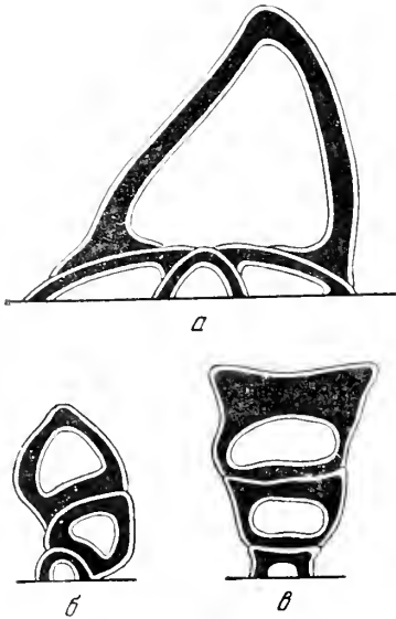
Рис. 1. Схема строения стенки камер миллиолид. a — Quinqueloculina ; б — Sigmoilina ; в — Spiroloculina .
