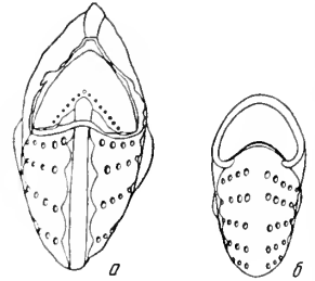
Фиг. 3. Дырчатое устье (а) Canalifera eichwaldi (Bogd.) и щелевидное устье (б) Canalifera clara Kr. \times 40 .
