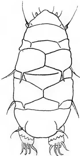
Fig. 45. — Echiniscus spec.
