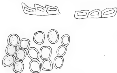
Fig. 75: Accidium Lantanae .
