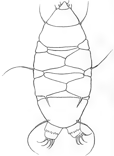
Fig. 46. — Echiniscus spec.
