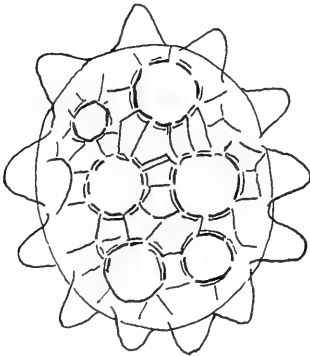
Fig. 43. — Macrobiotus spec.
