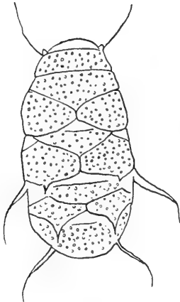
Fig. 44. — Echiniscus spec.
