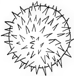
Fig. 42. — Macrobiotus spec.
