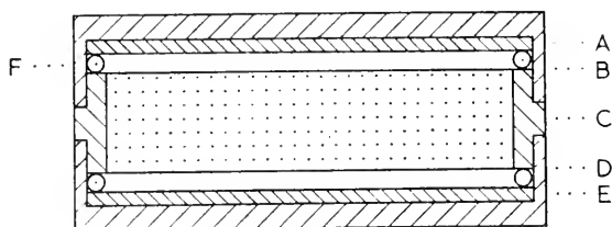
FIG. 1b. The diffusion cell.
