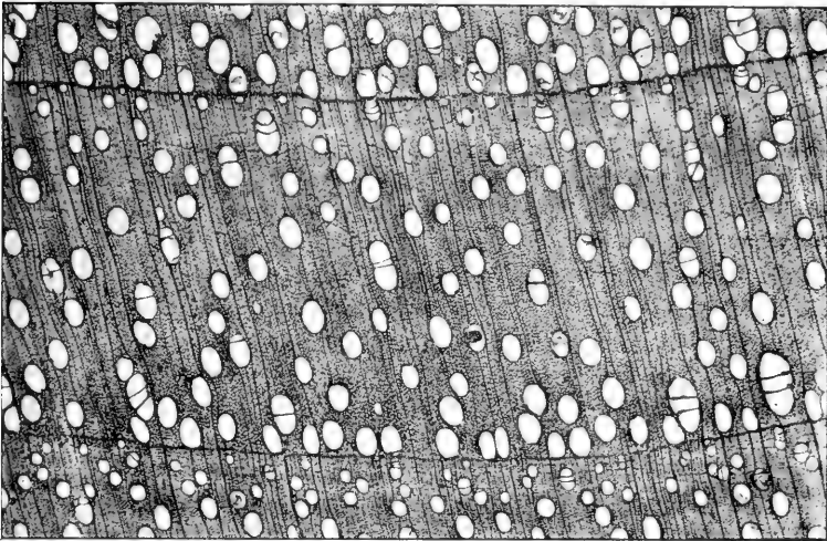
FIG. 36.—Transverse section of Butternut ( Juglans cinerea ).
