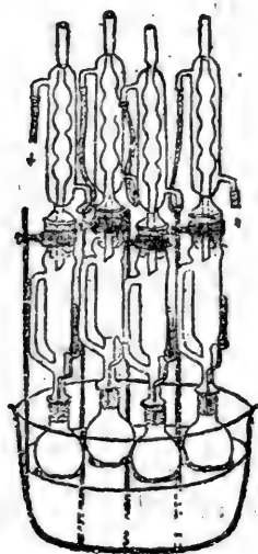
图 2 索氏提取器
