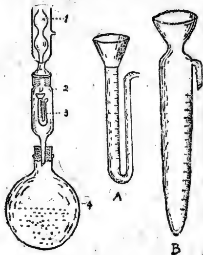
圖 3 測定芳香油的裝置
