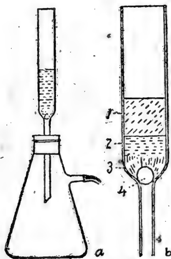
图 1 玻璃棉过滤器的装置
