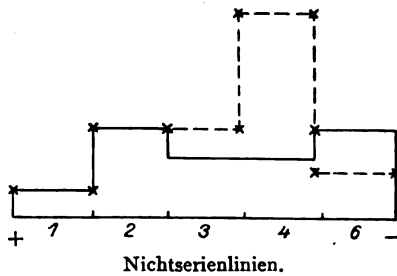
B. Quecksilberlinien.
