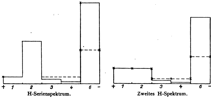
A. Wasserstofflinien.
