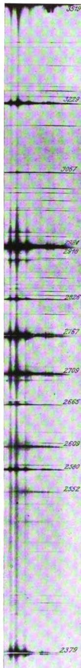
Tl-Spektrum.
