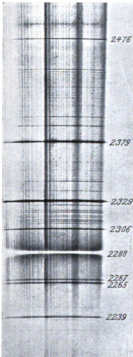
Cd-Spektrum.
