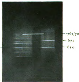
4a: \left\{ \begin{matrix} \text{Tageslicht, Funkenlicht} \\ \text{Röntgenstrahlen} \end{matrix} \right\} + \text{Druck.}
