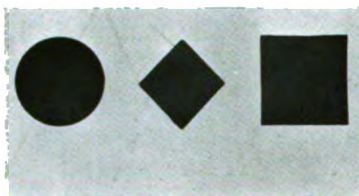
4a: \left\{ \begin{matrix} \text{Tageslicht, Funkenlicht} \\ \text{Röntgenstrahlen} \end{matrix} \right\} + \text{Druck.}
