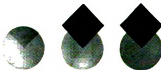
3a: Funkenlicht + Röntgenstrahlen
