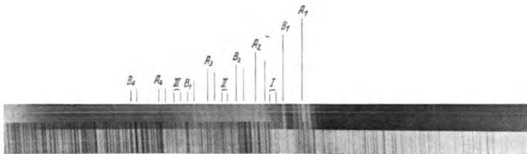
b) Benzaldehyd.
