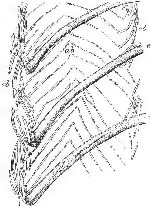
Figur 3. Reconstruction der zu einer Rumpfrippe von Kadaliosaurus priscus gehörigen abdominalen Ossifikationsstreifen und deren Verbindungsstücke.
