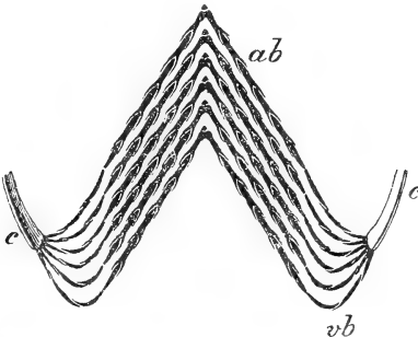
Figur 3. Reconstruction der zu einer Rumpfrippe von Kadaliosaurus priscus gehörigen abdominalen Ossifikationsstreifen und deren Verbindungsstücke.
