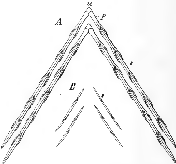
Figur 1. Abdominale Ossificationsstreifen von Kadalisaurus priscus .
