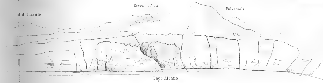
Der grosse Central Krater (Campo di Annibale) ges. aus d. Gegend v. Tusculum.
