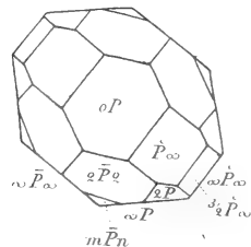
Fig. 31-36. Krystalle von grünem wasserhaltigen Enstatit. Oedegarden.
