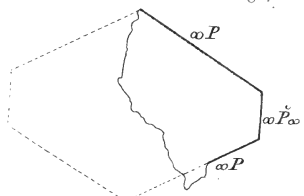
Fig. 26. Durchschnitt (nach oP ) 2\bar{P}_\infty eines Kjerulfinkrystalls.
