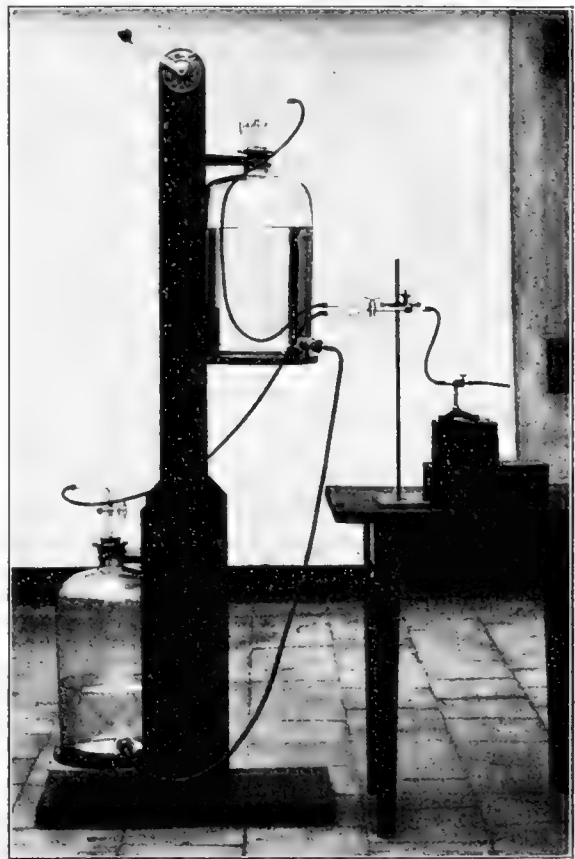
Fig. 8. Der Aspirator.
