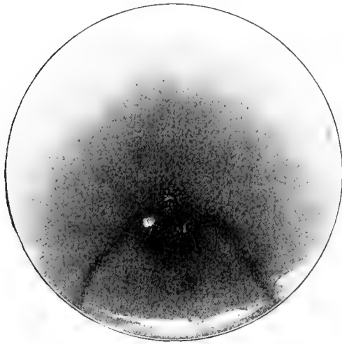
Fig. 3. Phormidium autumnale .
