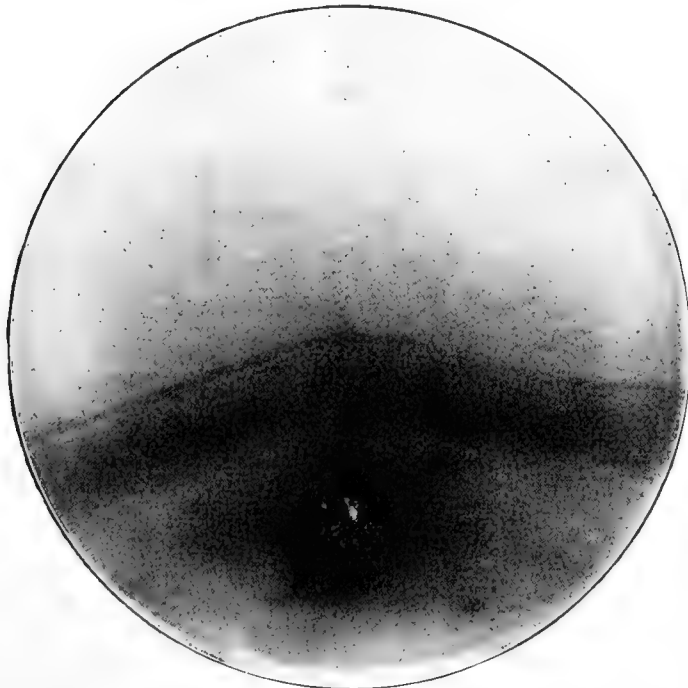
Fig. 4. Phormidium autumnale .
